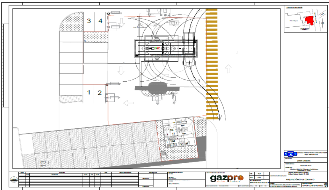
FIGURA 24. PLANO GENERAL DEL PROYECTO. ESPECIFICACIONES EN ANEXO 10
