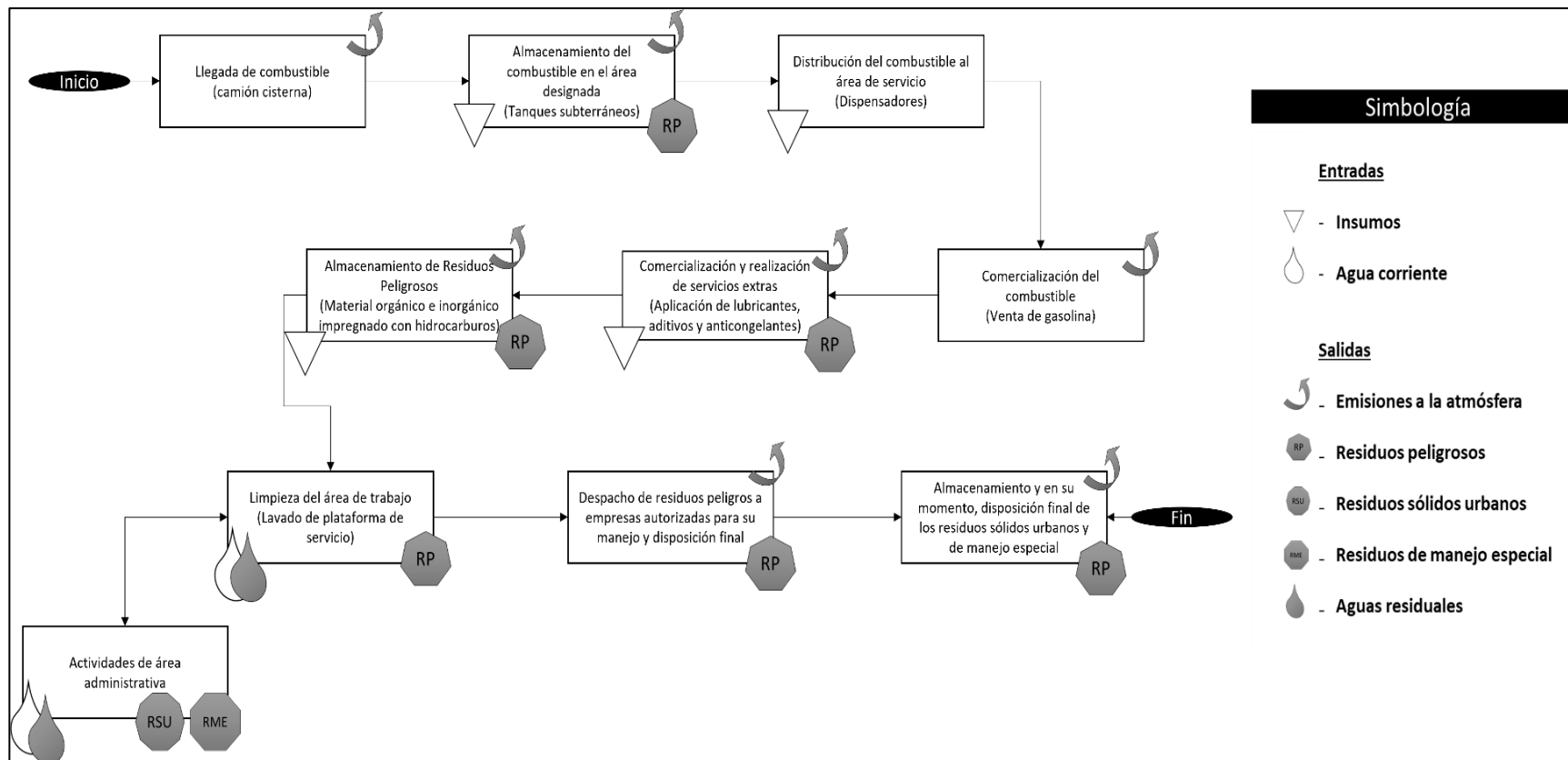
FIGURA 13. DIAGRAMA DE PROCESOS PARA LA COMERCIALIZACIÓN DE HIDROCARBUROS E IDENTIFICACIÓN DE SUS EMISIONES, DESCARGAS Y GENERACIÓN DE RESIDUOS
