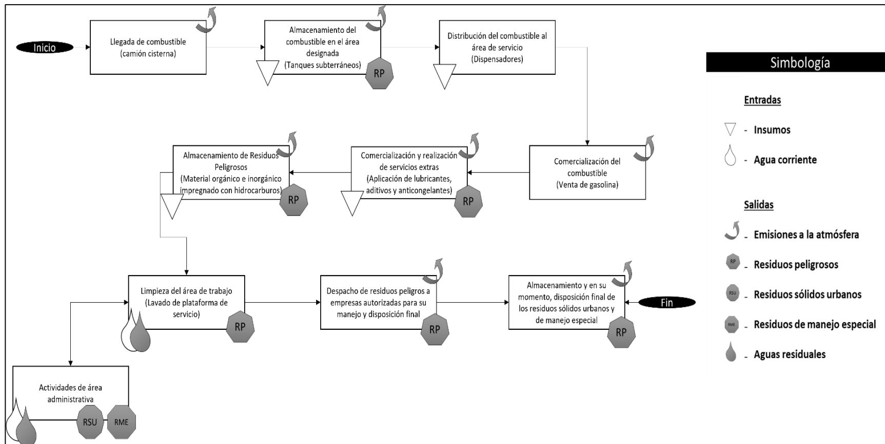
FIGURA 11. DIAGRAMA DE PROCESOS PARA LA COMERCIALIZACIÓN DE HIDROCARBUROS E IDENTIFICACIÓN DE SUS EMISIONES, DESCARGAS Y GENERACIÓN DE RESIDUOS
