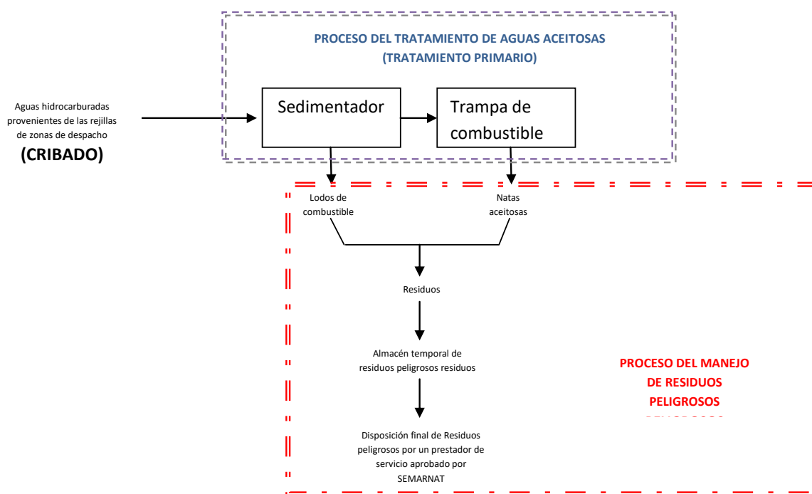
Figura 14. Proceso de tratamiento de aguas aceitosas
