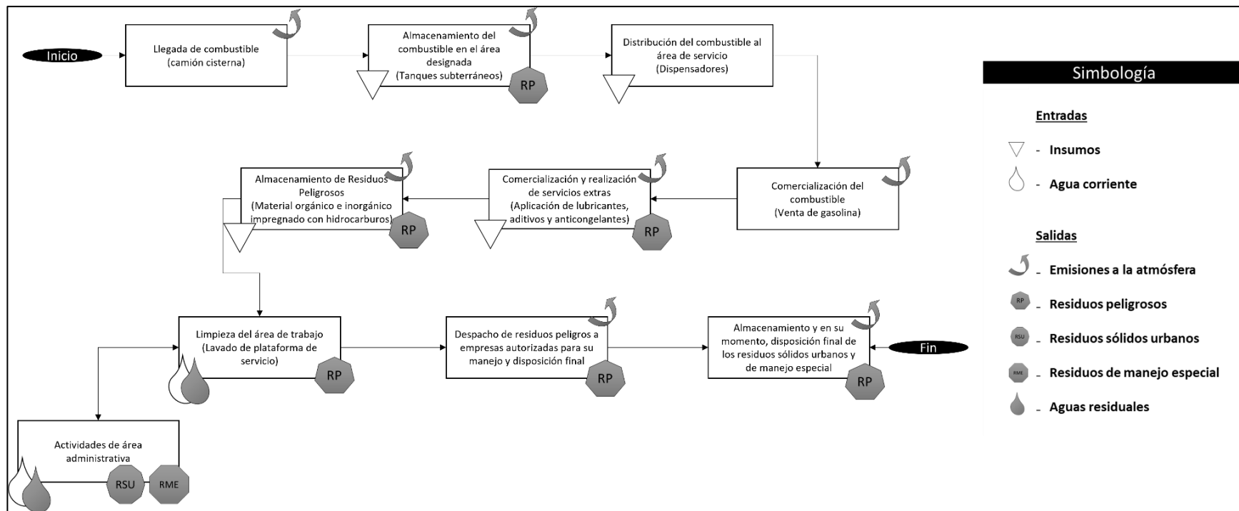
FIGURA 12. DIAGRAMA DE PROCESOS PARA LA COMERCIALIZACIÓN DE HIDROCARBUROS E IDENTIFICACIÓN DE SUS EMISIONES, DESCARGAS Y GENERACIÓN DE RESIDUOS
