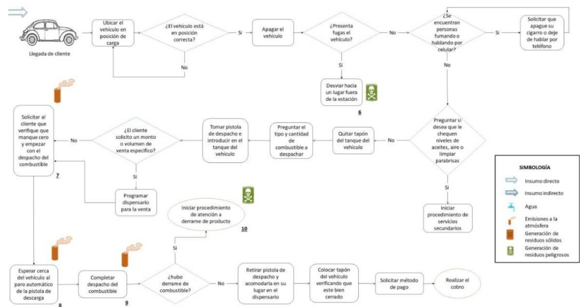
DIAGRAMA DE PROCEDIMIENTO DE DESPACHO DE COMBUSTIBLE
