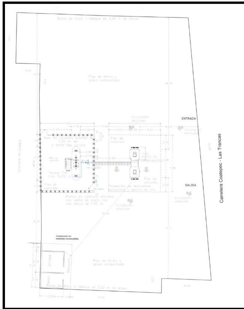
Ilustración 2 Plano civil de la Estación de Gas L.P. para Carburación
