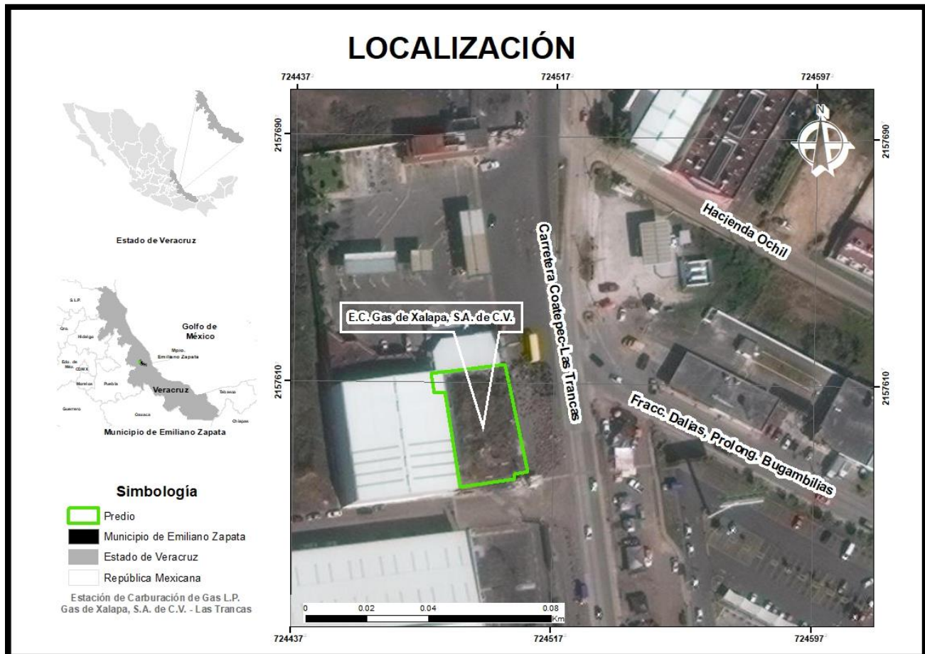
Ilustración 1 Ubicación regional y local de la Estación de Gas L.P. para Carburación dentro del municipio de Emiliano Zapata
