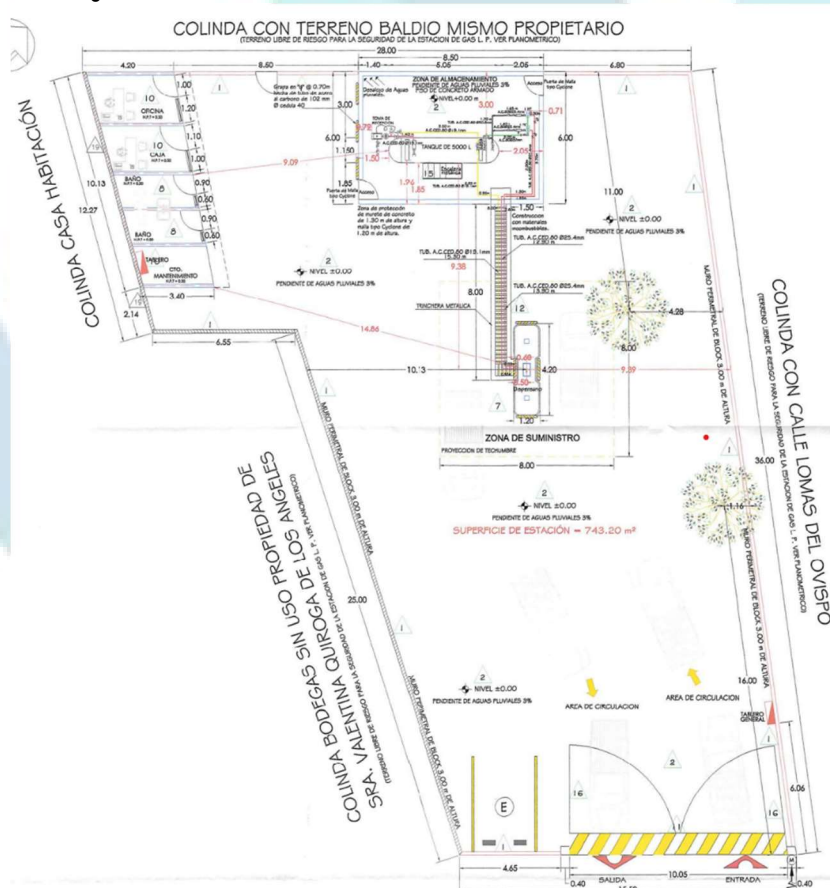
Imagen 13. Plano Civil del proyecto de la Estación de Gas L.P. para Carburación.
