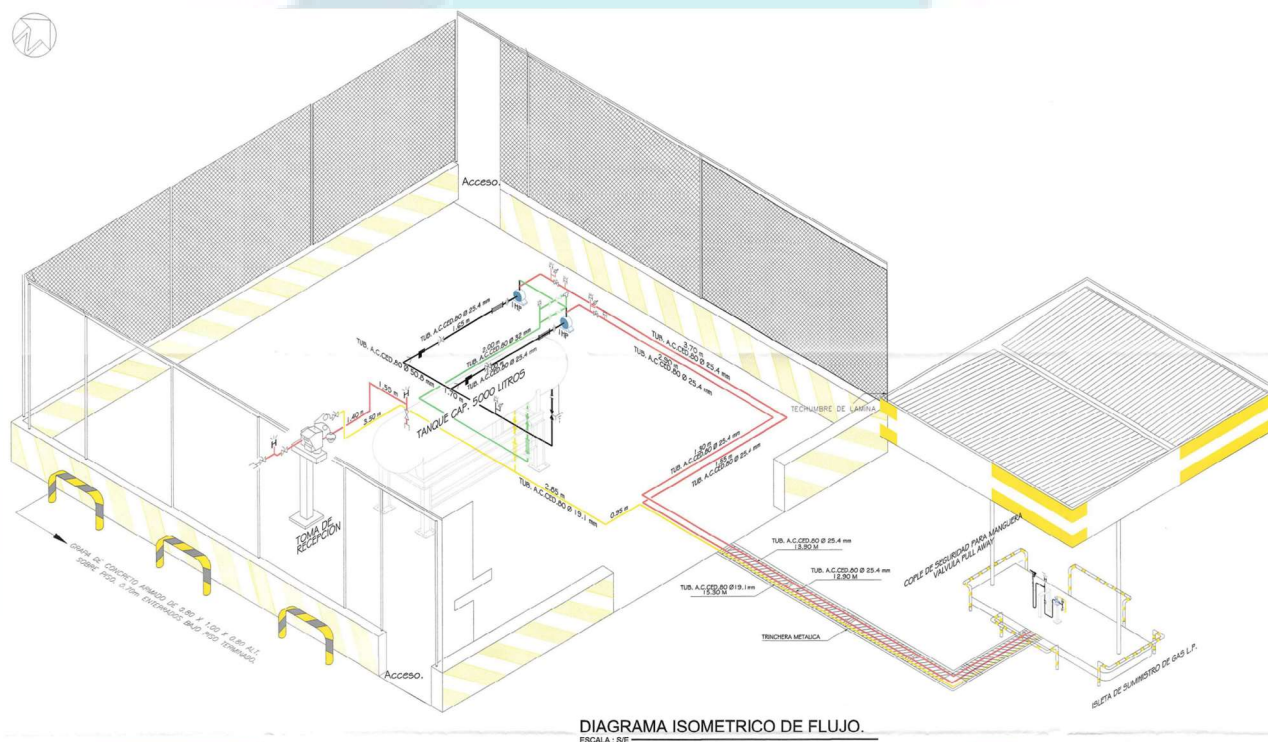
Imagen 11. Plano Mecánico del proyecto de la Estación de Gas L.P. para carburación
