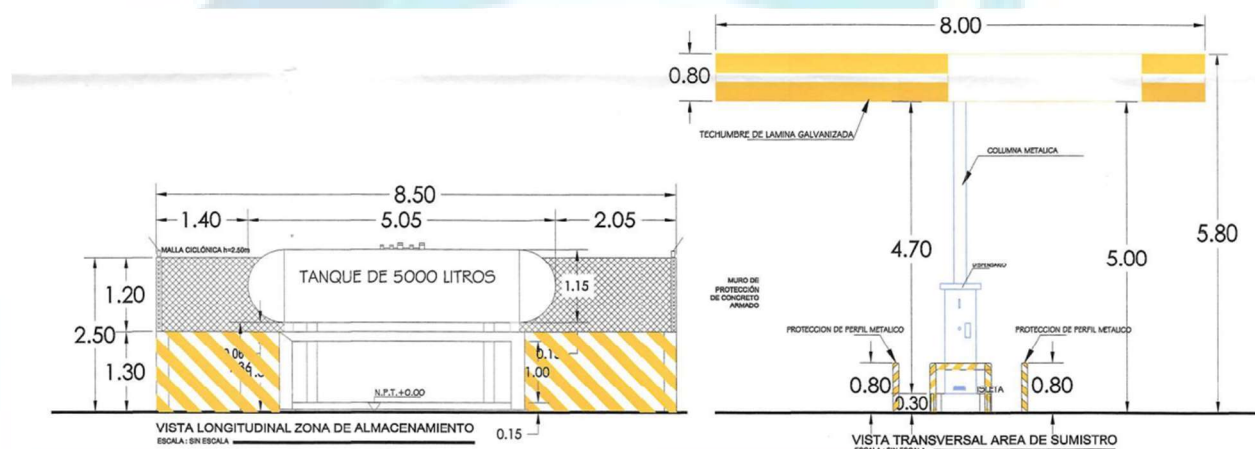
Imagen 14. Vista Longitudinal del Tanque de Almacenamiento.
