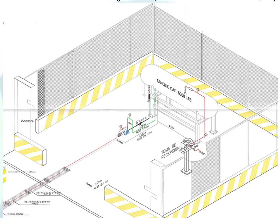
Plano Mecánico del proyecto de la Estación de Gas L.P. para carburación
