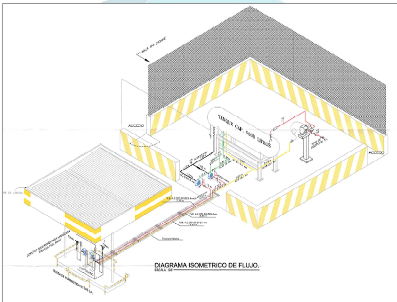
Imagen 11. Plano Mecánico del proyecto de la Estación de Gas L.P. para carburación
