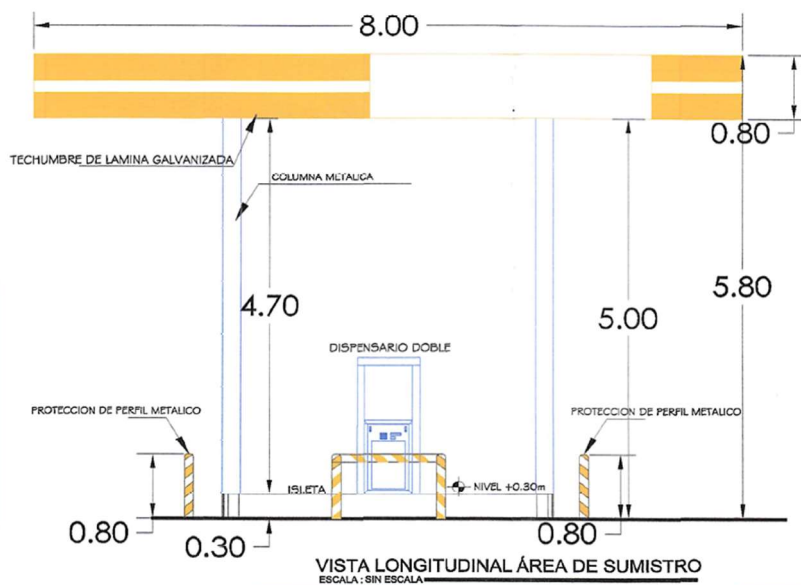
Imagen 14. Toma de suministro de la Estación de Gas L.P. para Carburación.
