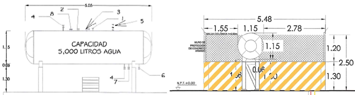
Imagen 13. Vista Longitudinal del Tanque de Almacenamiento.
