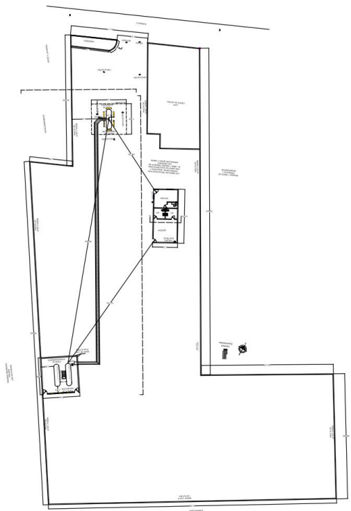
Figura III.1.b)-2. Plano Proyecto Civil
