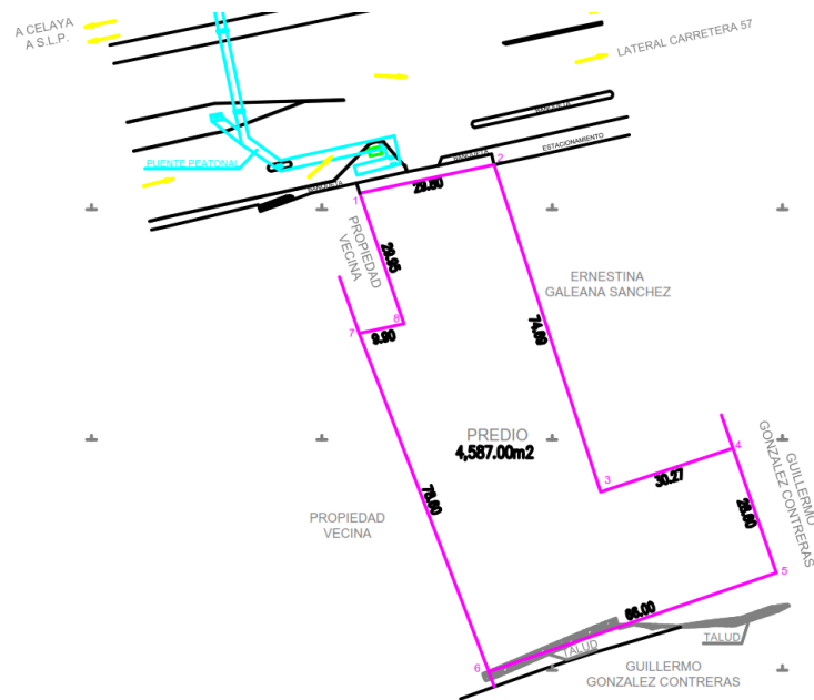
Figura III.1.b)-1 Plano topográfico
