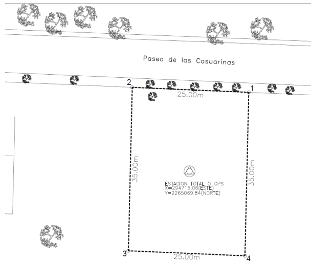
Figura III.1.b)-1 Plano Topográfico
