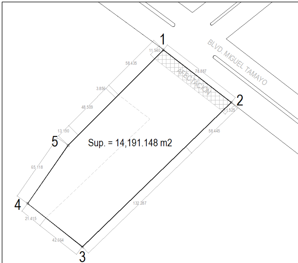
Figura 7. Polígono de la Estación de Servicio.
