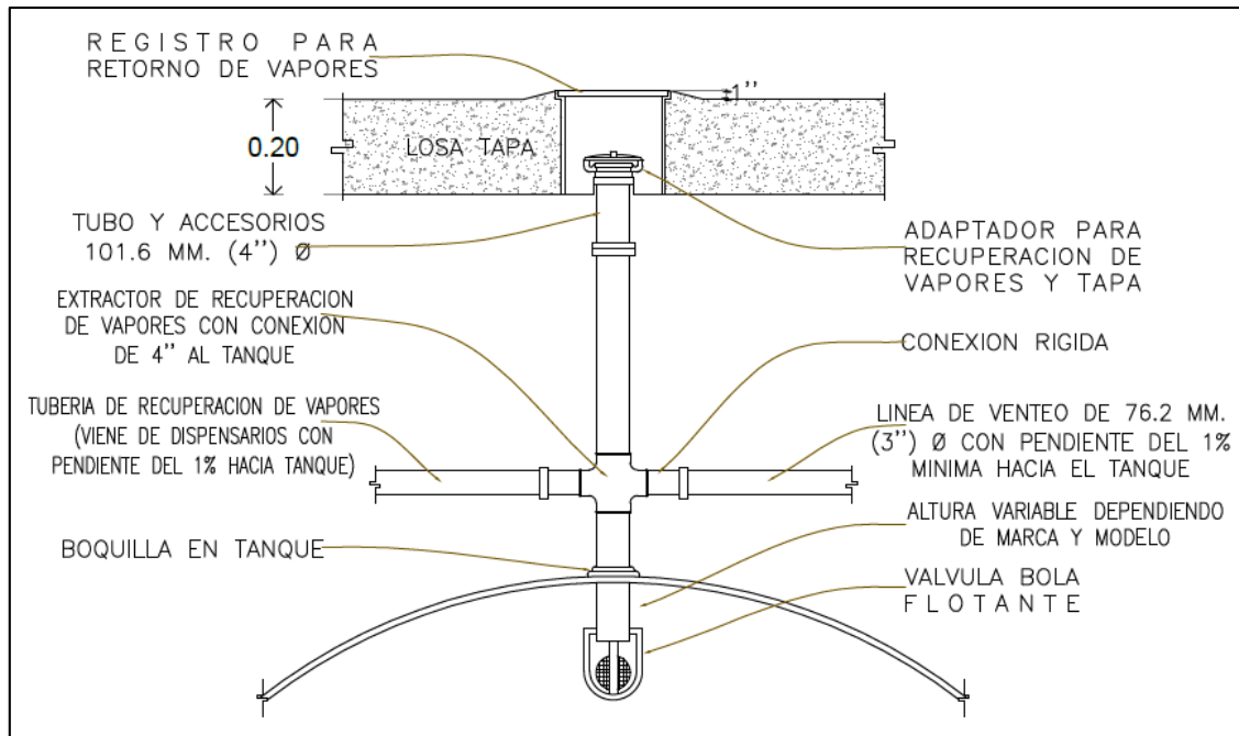
Figura 18. Detalles del sistema recuperador de vapores en los tanques de almacenamiento.
