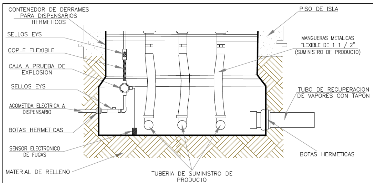
Figura 19. Detalles del sistema recuperador de vapores en las bombas de despacho.
