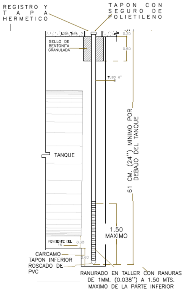
Figura 20. Características del pozo de observación.
