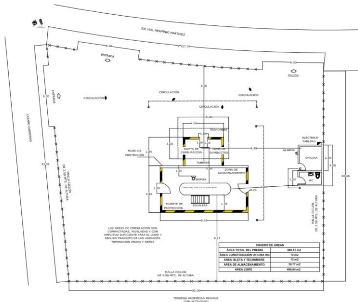
Figura I.1.2.-2. Plano Proyecto Civil
