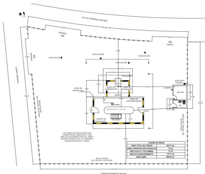
Figura III.1.b)-2. Plano Proyecto Civil
