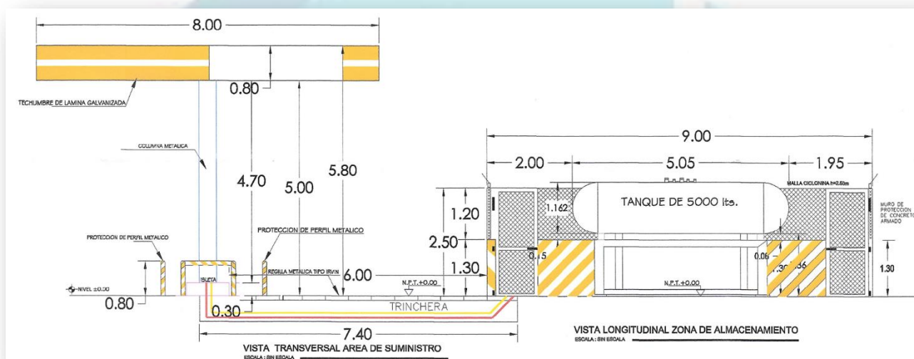
Imagen 14. Vista Longitudinal del recipiente de almacenamiento.
