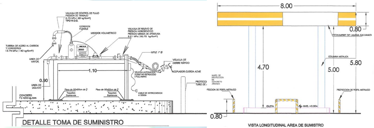
Imagen 15. Toma de suministro de la Estación de Gas L.P. para Carburación.
