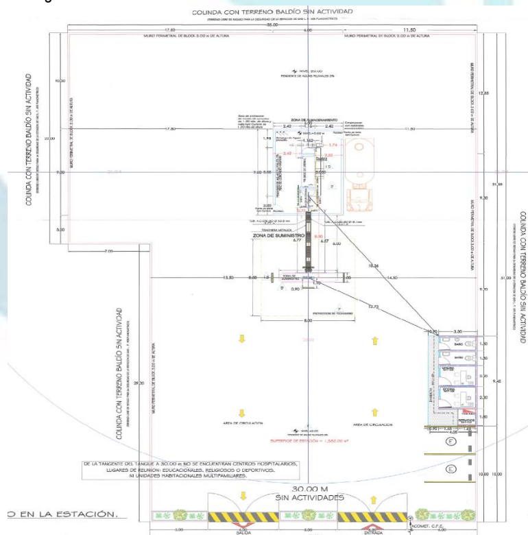
Imagen 13. Plano Civil del proyecto de la Estación de Gas L.P. para Carburación.
