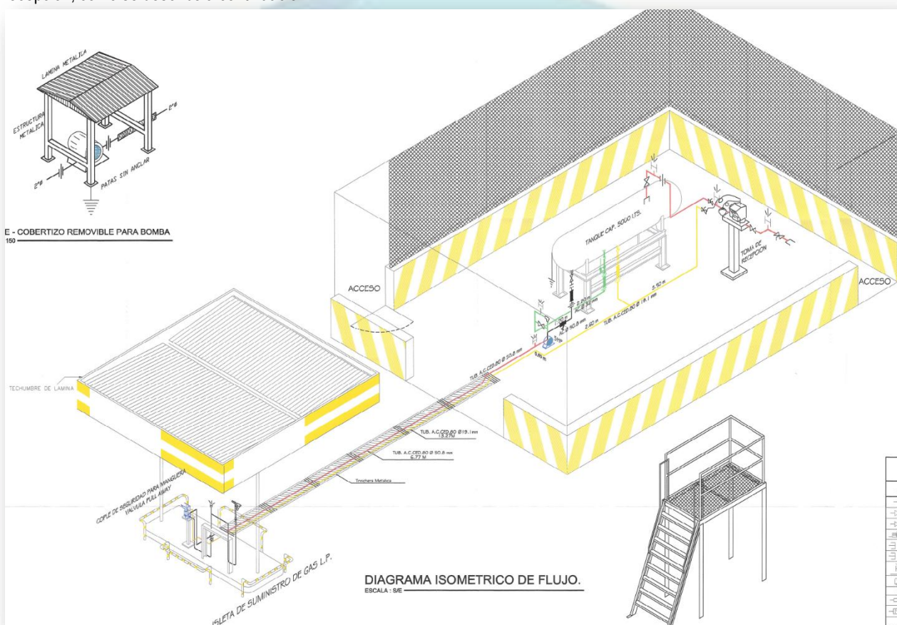
Imagen 11. Plano Mecánico del proyecto de la Estación de Gas L.P. para carburación
