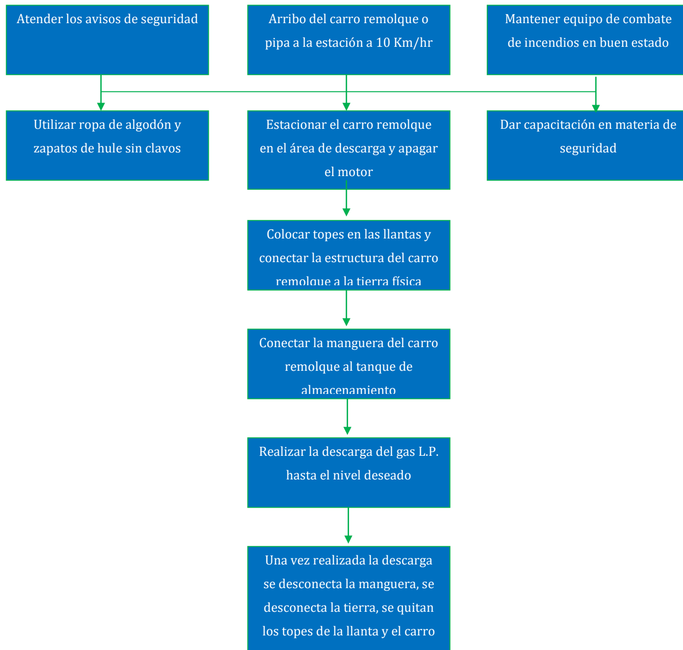
Figura 13. Descarga de Gas L.P.
