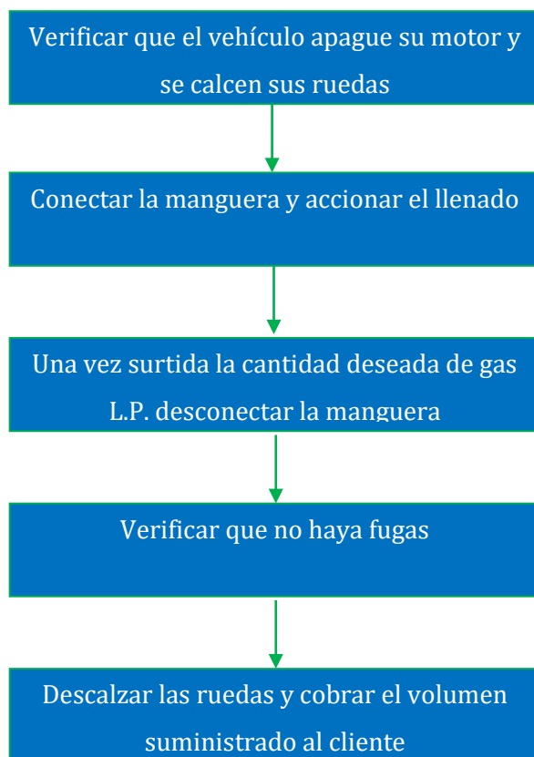
Figura 14. Operación de Trasiego
