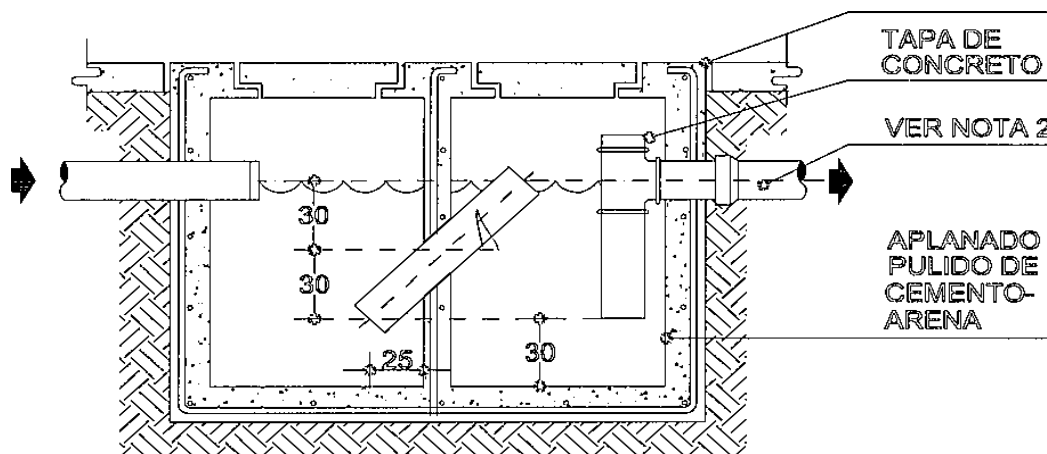
IMAGEN 8. TRAMPA DE COMBSUTIBLES
