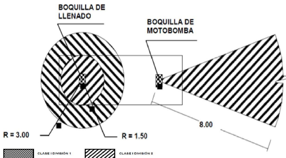
IMAGEN 5 CLASIFICACIÓN DE ÁREA PELIGROSA TANQUE DE ALMACENAMIENTO
