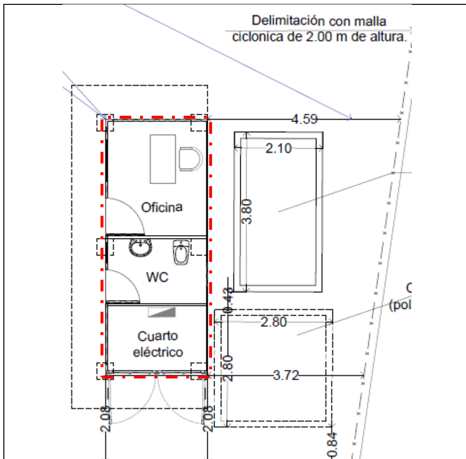
FIGURA III.1.3.2. EDIFICIO DE OFICINA Y SERVICIOS SANITARIOS DE LA ESTACIÓN | FUENTE: PLANO DEL PROYECTO PLANOMÉTRICO Y PLANO DEL PROYECTO CIVIL | ANEXO 3 EXPEDIENTE TÉCNICO DEL PROYECTO
