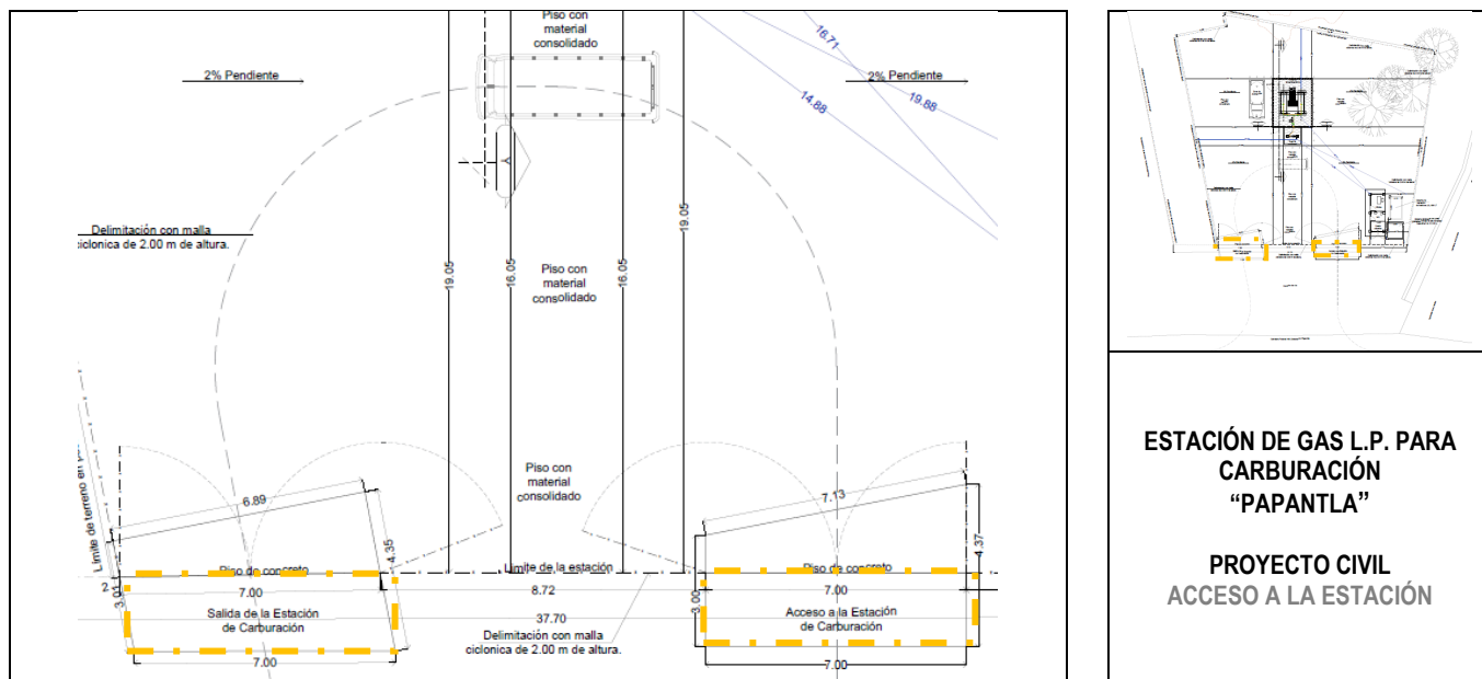
FIGURA III.1.3.1. ACCESO A LA ESTACIÓN | FUENTE: PLANO DEL PROYECTO PLANOMÉTRICO | ANEXO 3 EXPEDIENTE TÉCNICO DEL PROYECTO
