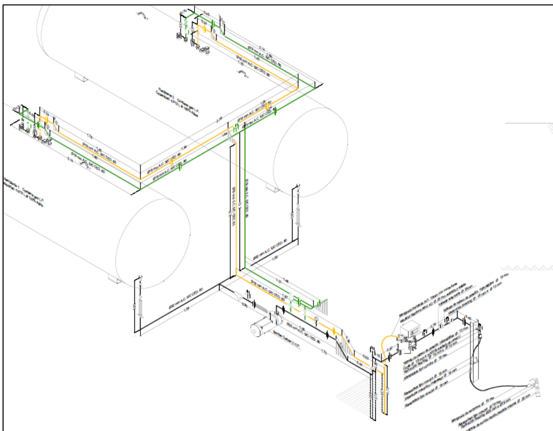
FIGURA III.1.3.6. DIAGRAMA ISOMÉTRICO DE LA INSTALACIÓN DE ALMACENAMIENTO-IMPULSIÓN Y TRANSPORTE DE GAS LP EN LA ESTACIÓN | FUENTE: PLANO DEL PROYECTO MECÁNICO | ANEXO 3 EXPEDIENTE TÉCNICO DEL PROYECTO
