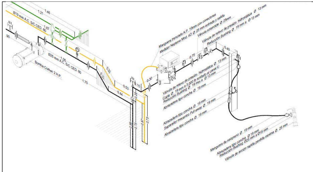
FIGURA III.1.3.7. DETALLE DE LA TOMA DE SUMINISTRO DE GAS LP DE LA ESTACIÓN | FUENTE: PLANO DEL PROYECTO MECÁNICO | ANEXO 3 EXPEDIENTE TÉCNICO DEL PROYECTO
