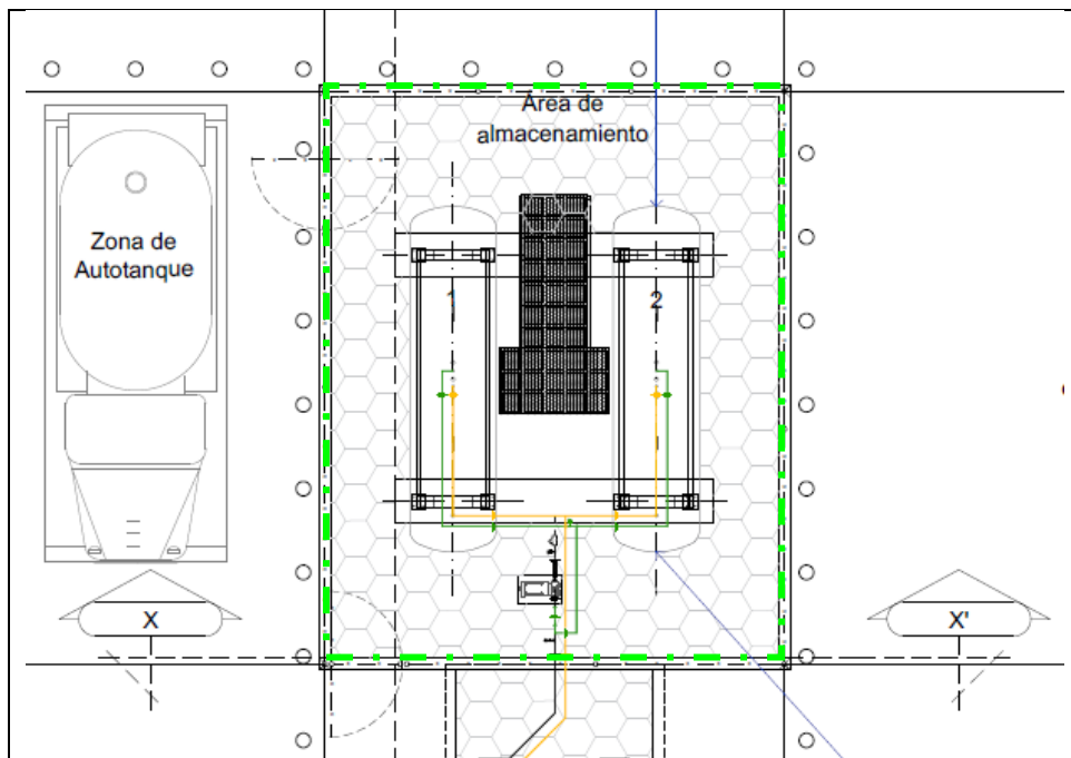
FIGURA III.1.3.3. ÁREA DE ALMACENAMIENTO DE LA ESTACIÓN | FUENTE: PLANOMÉTRICO Y PLANO DEL PROYECTO CIVIL | ANEXO 3 EXPEDIENTE TÉCNICO DEL PROYECTO
