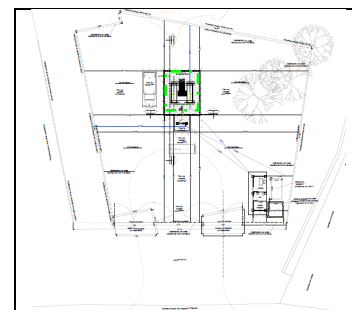
ESTACIÓN DE GAS L.P. PARA CARBURACIÓN “PAPANTLA” PROYECTO CIVIL ÁREA DE ALMACENAMIENTO DE GAS L.P. DE LA ESTACIÓN
