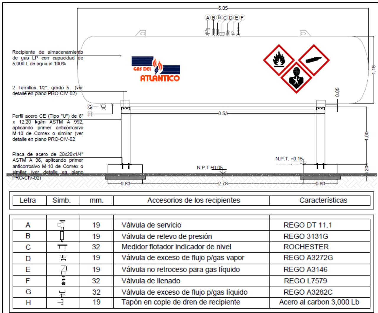
FIGURA III.1.3.4. LISTADO Y DISTRIBUCIÓN DE ACCESORIOS DEL TANQUE DE ALMACENAMIENTO FUENTE: PLANO DEL PROYECTO MECÁNICO | ANEXO 3 EXPEDIENTE TÉCNICO DEL PROYECTO
