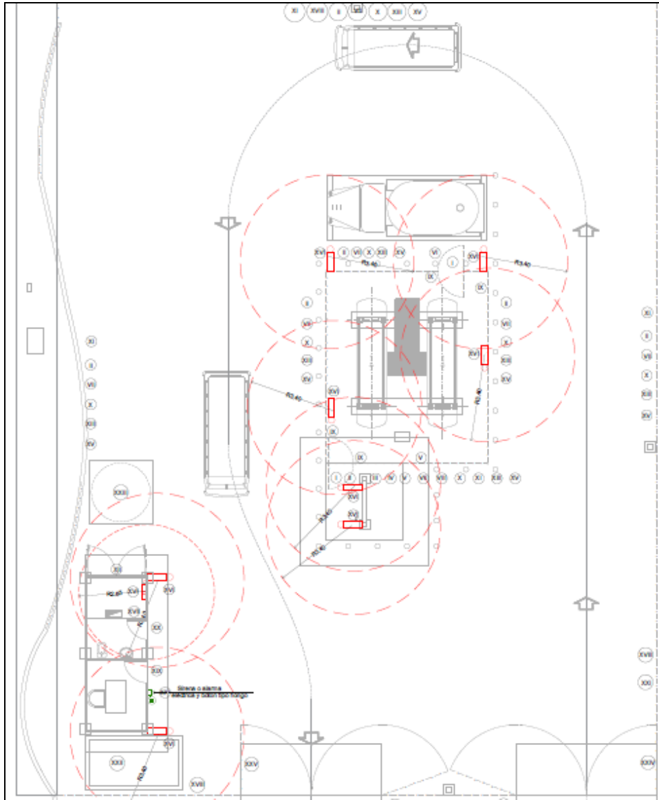
FIGURA III.1.3.8. DISTRIBUCIÓN DE EXTINTORES EN LA ESTACIÓN | FUENTE: PLANO DEL PROYECTO CONTRA INCENDIO ANEXO 3 EXPEDIENTE TÉCNICO DEL PROYECTO
