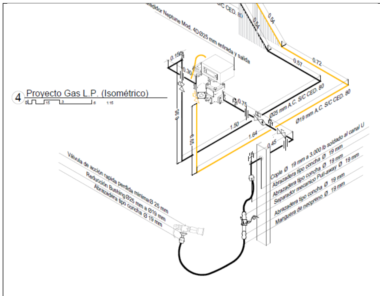
FIGURA III.1.3.7. DETALLE DE LA TOMA DE SUMINISTRO DE GAS LP DE LA ESTACIÓN | FUENTE: PLANO DEL PROYECTO MECÁNICO | ANEXO 3 EXPEDIENTE TÉCNICO DEL PROYECTO
