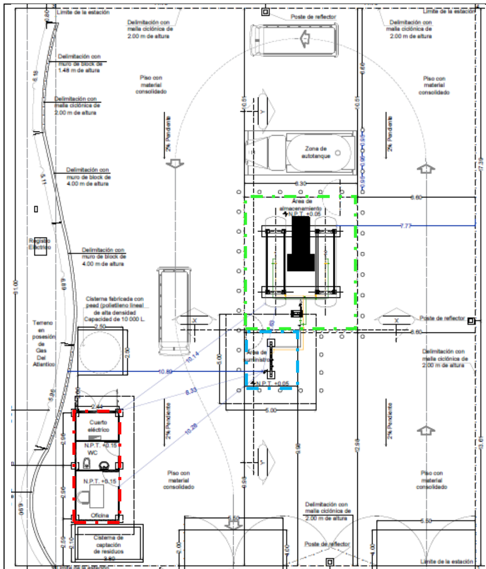
FIGURA III.1.2.1. PLANTA DE CONJUNTO PROSPECTIVA DEL PROYECTO CIVIL | FUENTE: PLANOMÉTRICO Y PLANO DEL PROYECTO CIVIL | ANEXO 3 EXPEDIENTE TÉCNICO DEL PROYECTO
