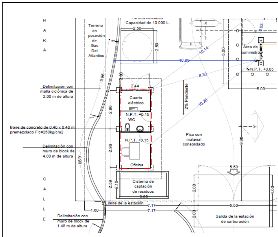
FIGURA III.1.3.2. EDIFICIO DE OFICINA Y SERVICIOS SANITARIOS DE LA ESTACIÓN | FUENTE: PLANO DEL PROYECTO PLANOMÉTRICO Y PLANO DEL PROYECTO CIVIL | ANEXO 3 EXPEDIENTE TÉCNICO DEL PROYECTO
