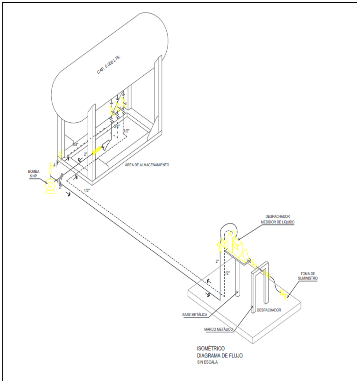
Ilustración 7 Diagrama de Tanque
