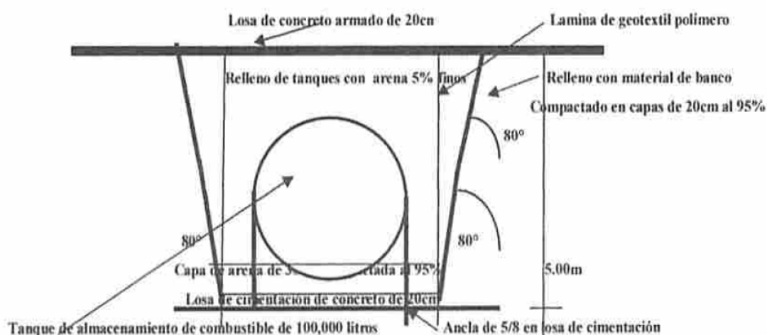
Croquis sin escala del sistema de excavación en zona de tanques
