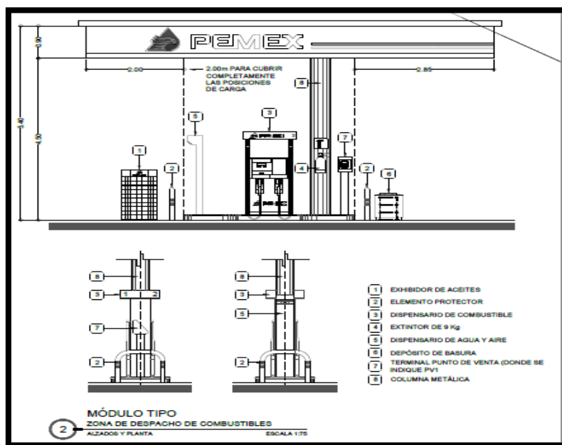
Imagen 10. Diagrama Tipo del Módulo de Abastecimiento.
