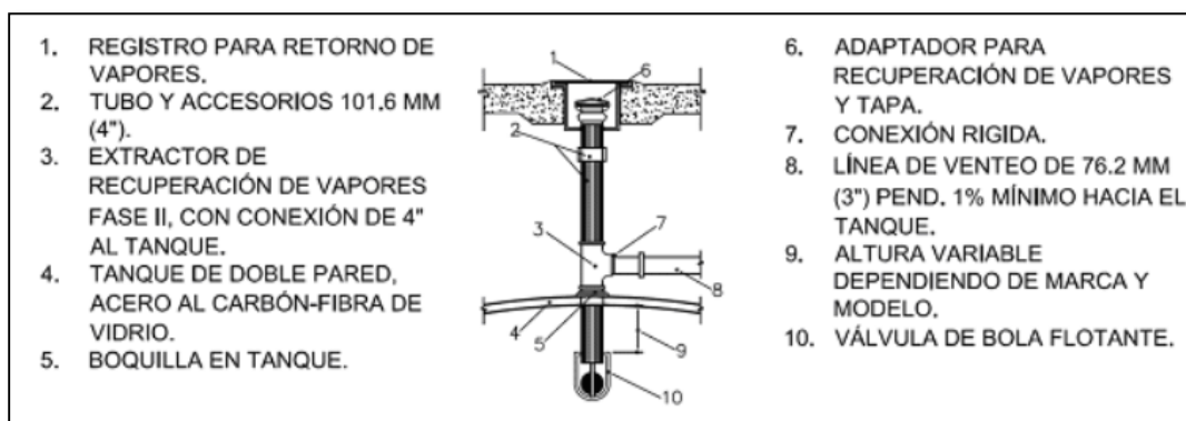
IMAGEN 6.- Sistema de recuperación de vapores
