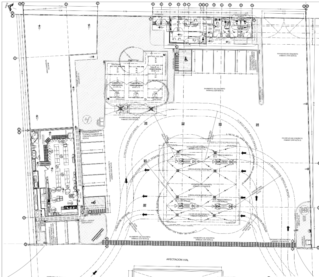
Figura 3. Plano de la estación de servicio.
