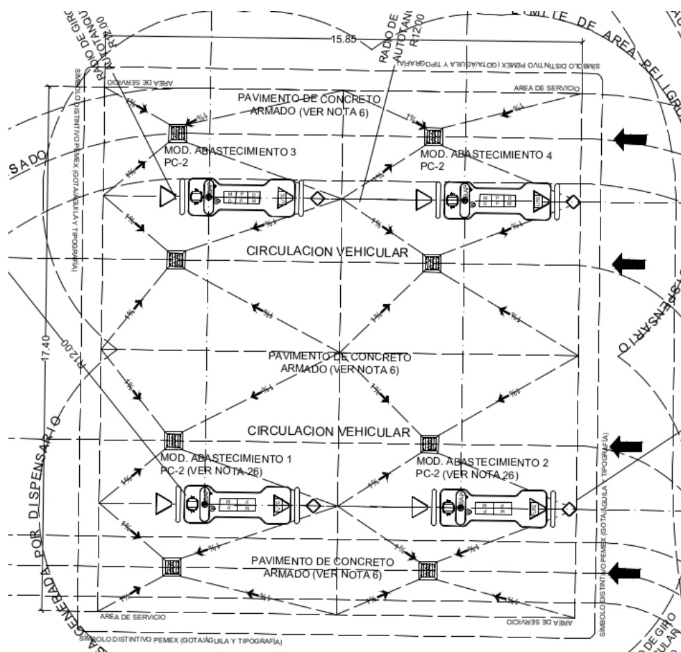
Figura 8. Área de dispensarios en la estación de servicio.
