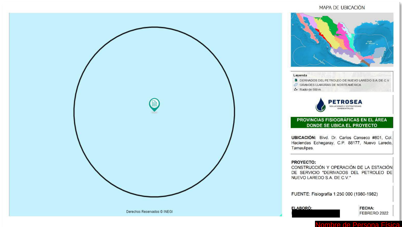
Figura 13. Provincias fisiográficas
