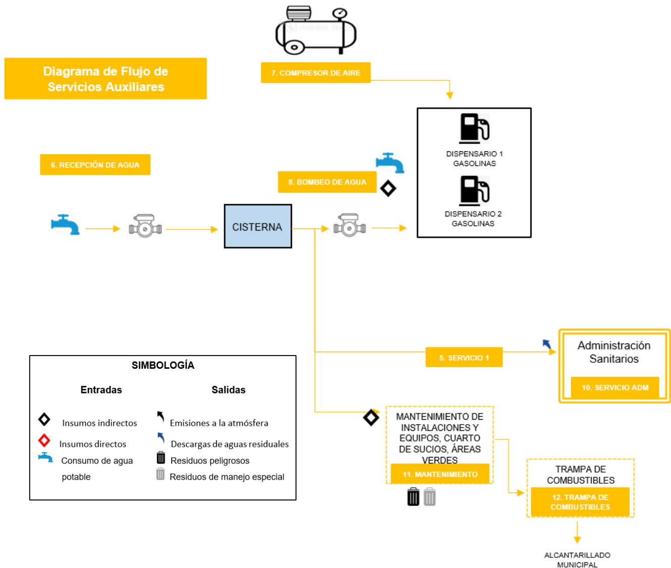
Figura 8. Diagrama de flujo de operaciones.
