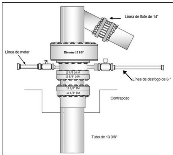
Figura 28 Arreglo del carrete de control y desviador de flujo 21 1/4" x 2M psi para Etapa 17 1/2" - Patriota-107 DEL
