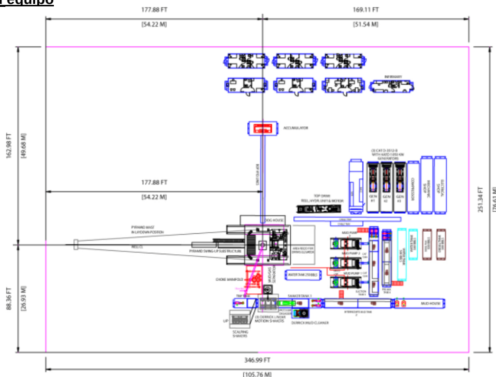
Figura 27 Diseño de arreglo de un equipo de perforación
