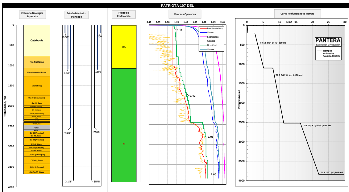
Figura 18 Estado mecánico propuesto Patriota-107DEL
