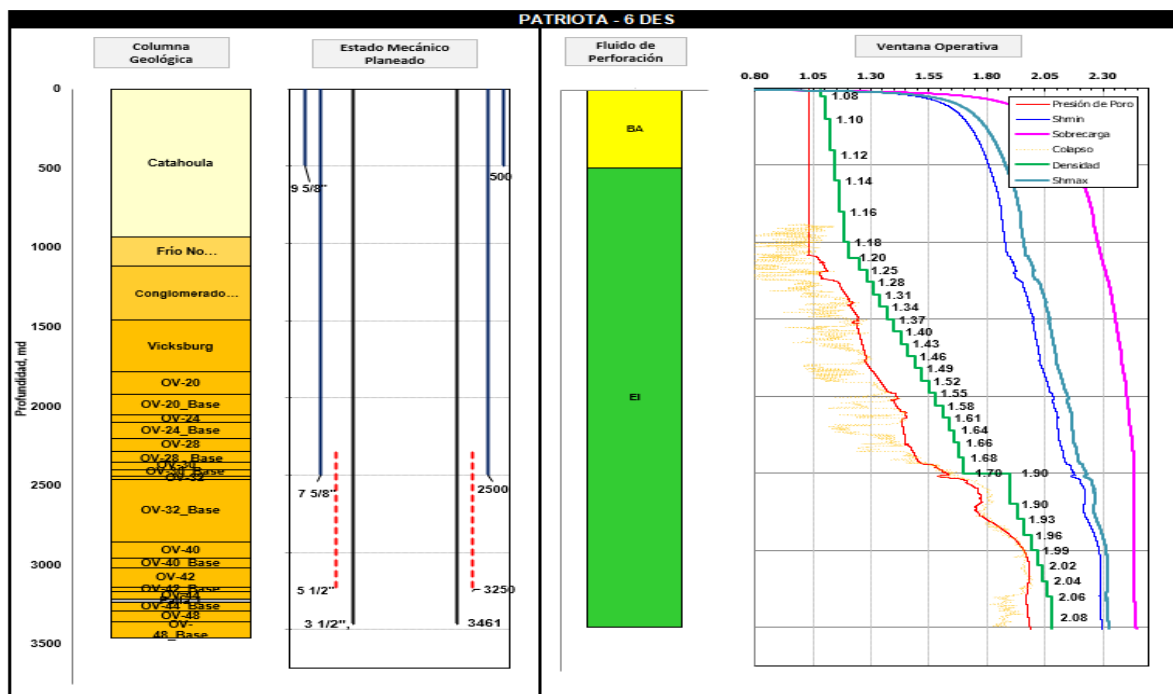
Figura 23 Estado Mecánico de Mitigación de Riesgo de la Localización Patriota-6 DES
