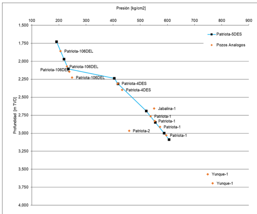
Figura 15 Gradiente de presión.
