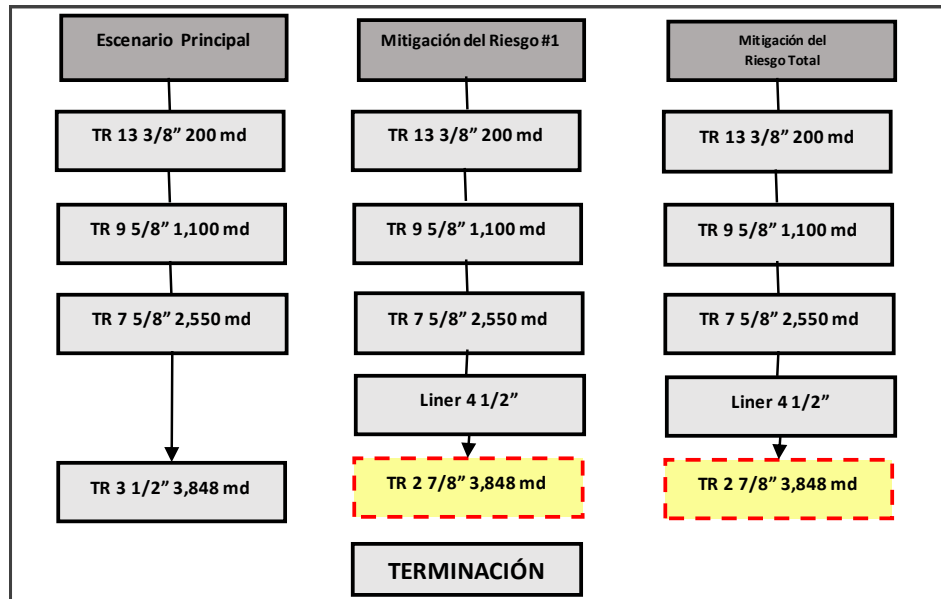
Figura 20 Escenarios de Mitigación de Riesgos para el proyecto pozo Patriota-107 DEL.
