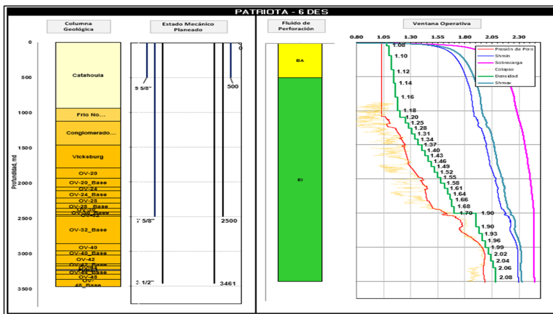
Figura 19 Estado mecánico propuesto Patriota-6DES
