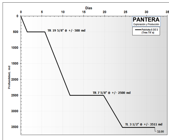
Figura 25 Gráfica de tiempo Vs. Profundidad
