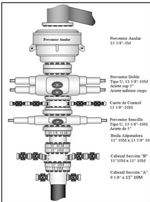
Figura 30 Arreglo de Preventor Esférico de 13 5/8" 5M con Ariete Superior Variable y Ariete Inferior Ciego, Carrete de Control de 13 5/8" 10M con Salidas Laterales de 3 1/16" 10M y Válvula Mecánica de 3 1/8", Brida de 3 1/16", Preventor Sencillo de 13 5/8" 10M y Cabezal 11" 10M para la Etapa 8 1/2" del Proyecto Pozo Patriota-107 DEL.
