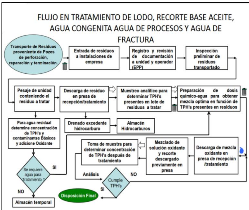
Figura 32 Diagrama de flujo del proceso de manejo de recortes
