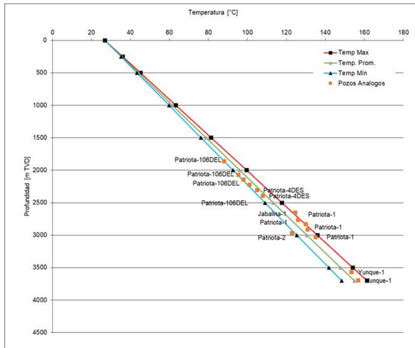
Figura 16 Gradiente de temperatura del pozo Patriota-107DEL
