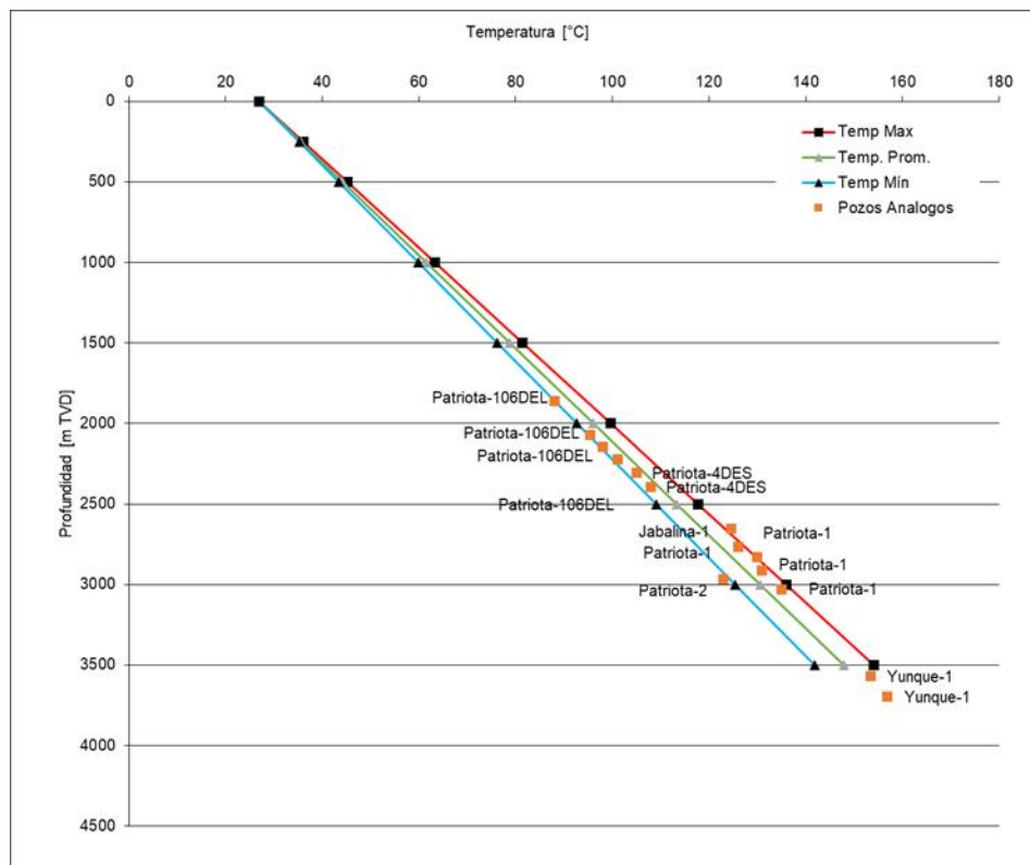
Figura 17 Gradiente de temperatura del pozo Patriota-6DES
