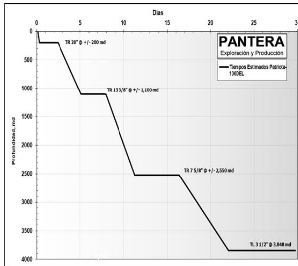
Figura 24 Gráfica de tiempo Vs. Profundidad
