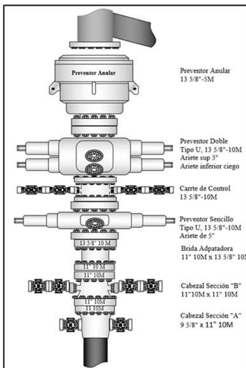
Figura 29 Arreglo 13 5/8" 10M y preventor anular 13 5/8" x 5M, para la etapa 12 1/4" del proyecto pozo Patriota-107 DEL
