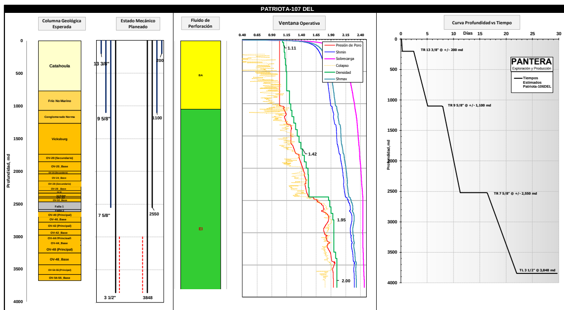
Figura 22 Estado Mecánico de Mitigación de Riesgo de la Localización Patriota-107 DEL
