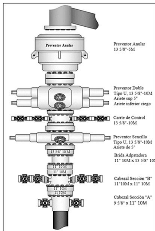
Figura 31 Arreglo 13 5/8\" 10M y preventor anular 13 5/8\" 5M.
