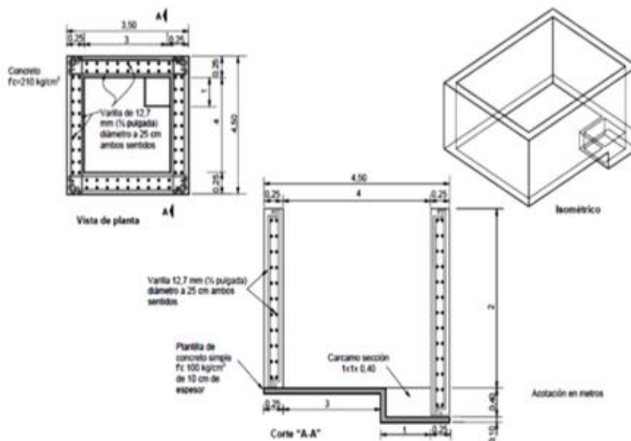
Figura 26 Diseño de contrapozo
