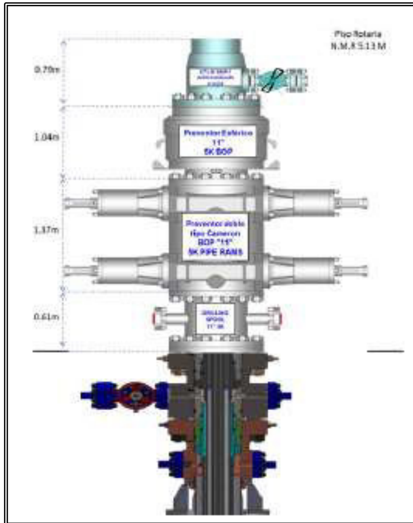
Figura III.1.2.5.3-1.- Conjunto de preventores para la fase 6 \frac{3}{4} ".
