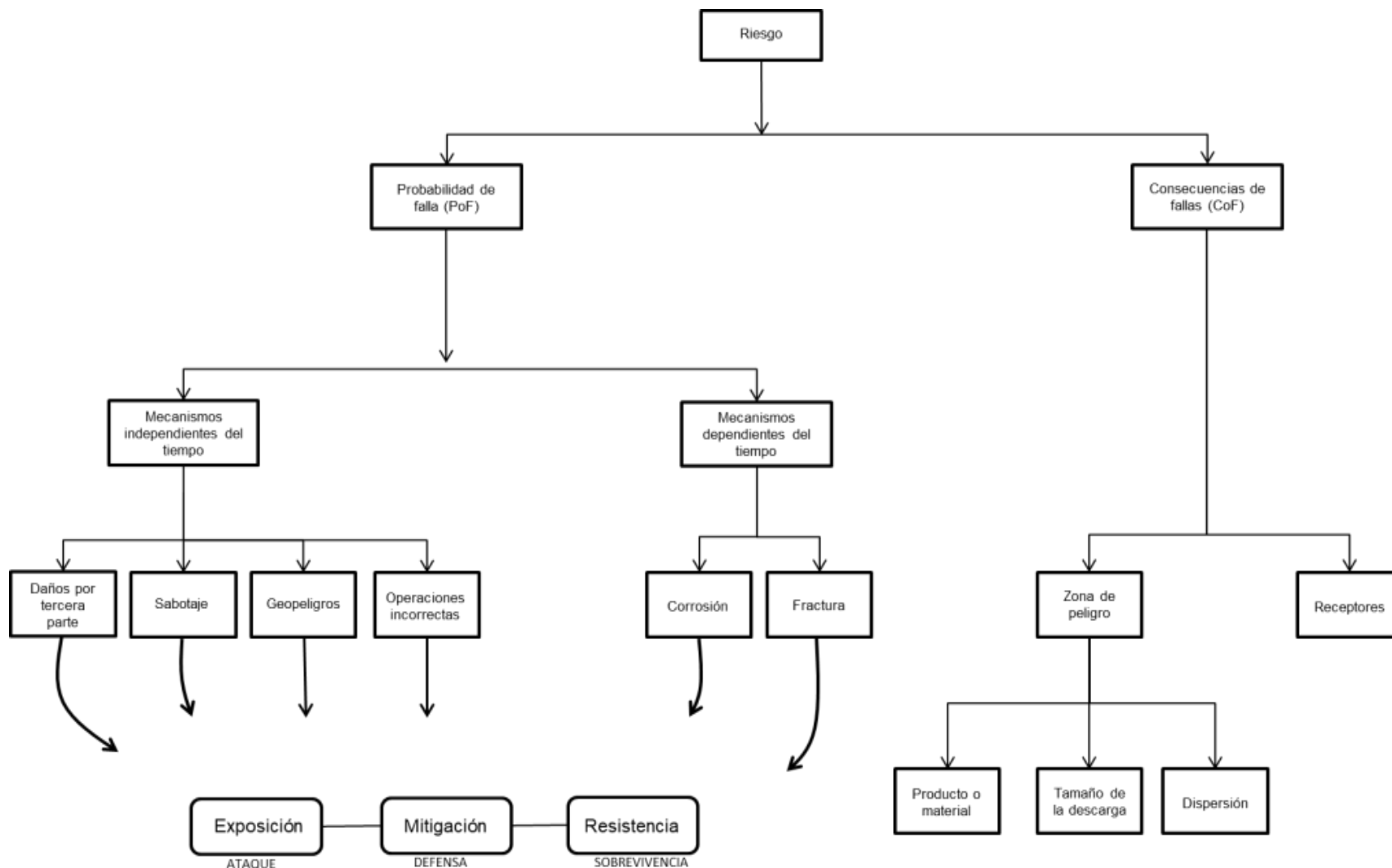
Figura IX.2. Modelo de riesgos en tuberías
