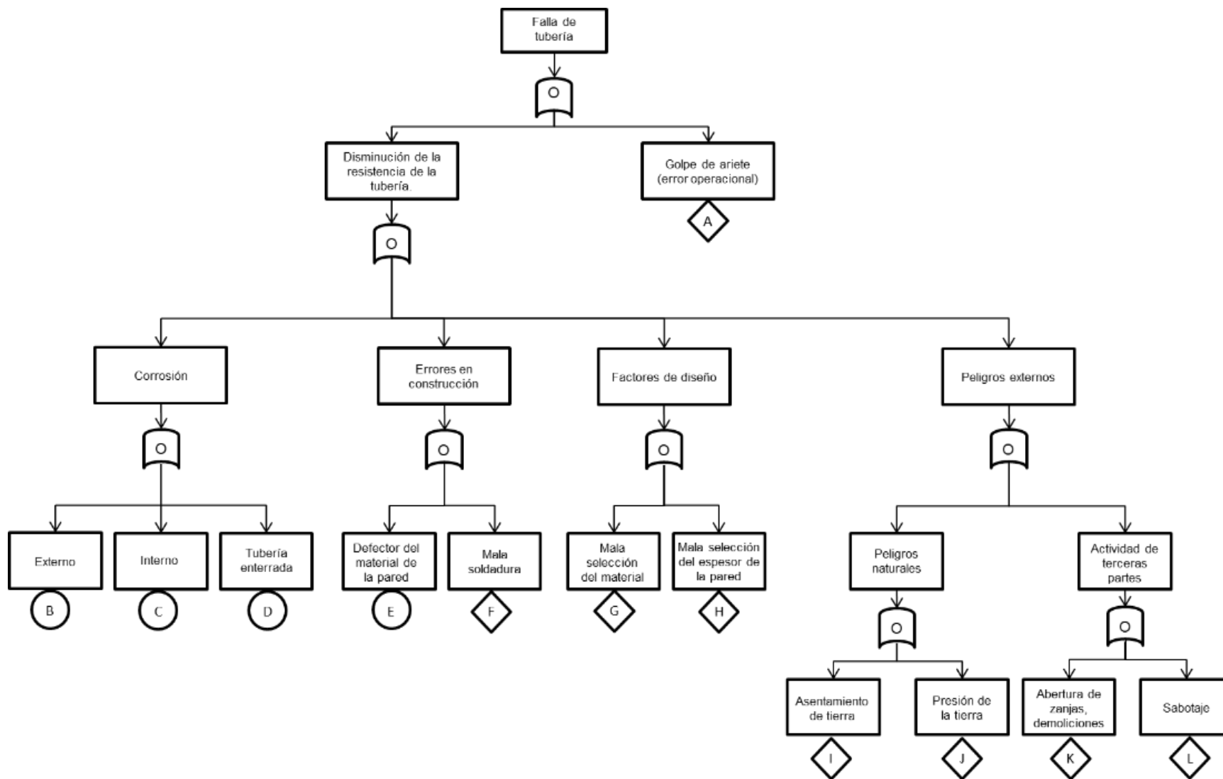
Figura IX.1. Árbol de causas de fallas en sistemas de tubería
