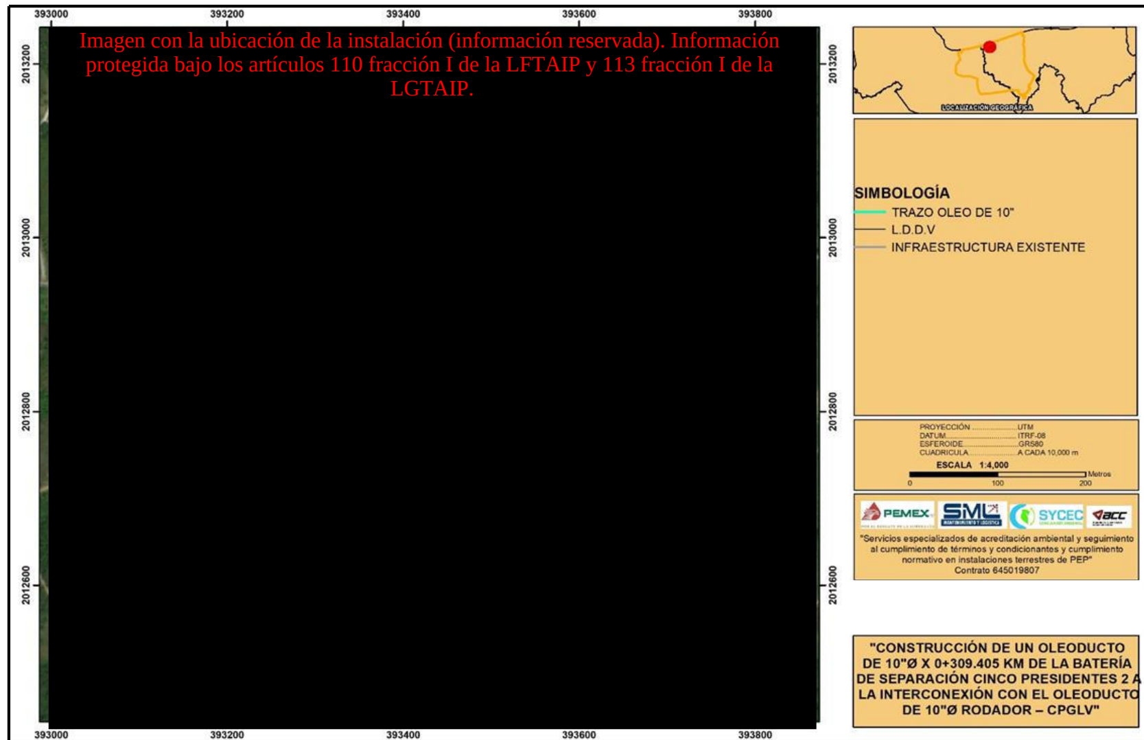
Figura IX.3. Mapa representativo del trazo del Oleoducto de 10"Ø x 0+309.405 km de la Batería de Separación Cinco Presidentes No. 2 a la Interconexión con el Oleoducto de 10"Ø Rodador-CPGLV.
