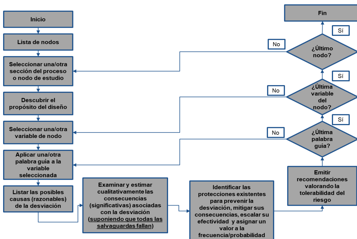
Diagrama IX.2. Protocolo de análisis de un HAZOP.
