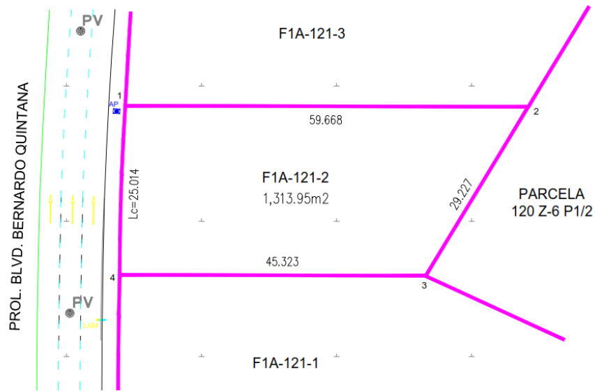
Figura I.1.2.-1. Plano topográfico
