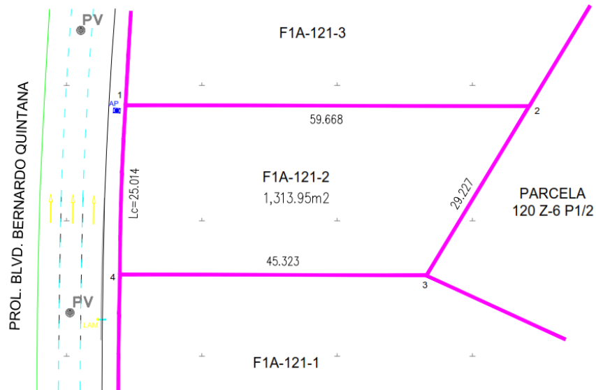
Figura III.1.b)-1 Plano topográfico
