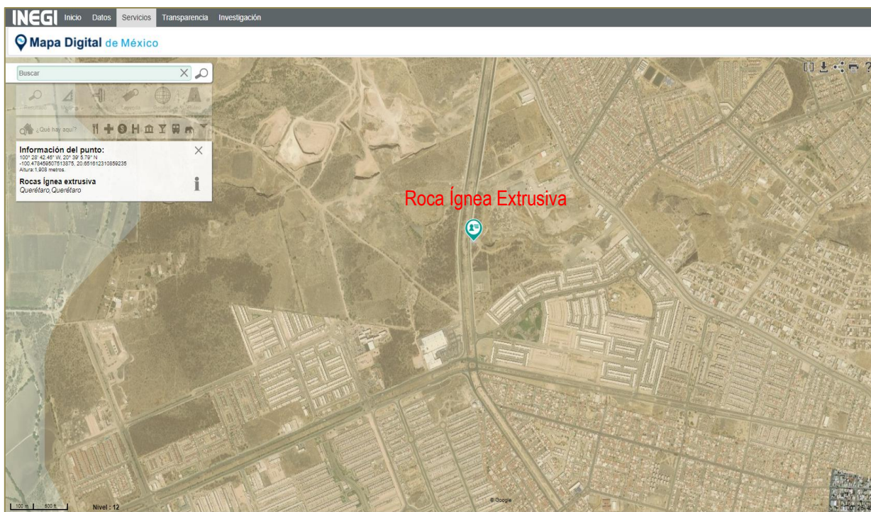
Figura III.4.d)-B2. Geología en el sitio del proyecto. Fuente: Mapa Digital de México.
