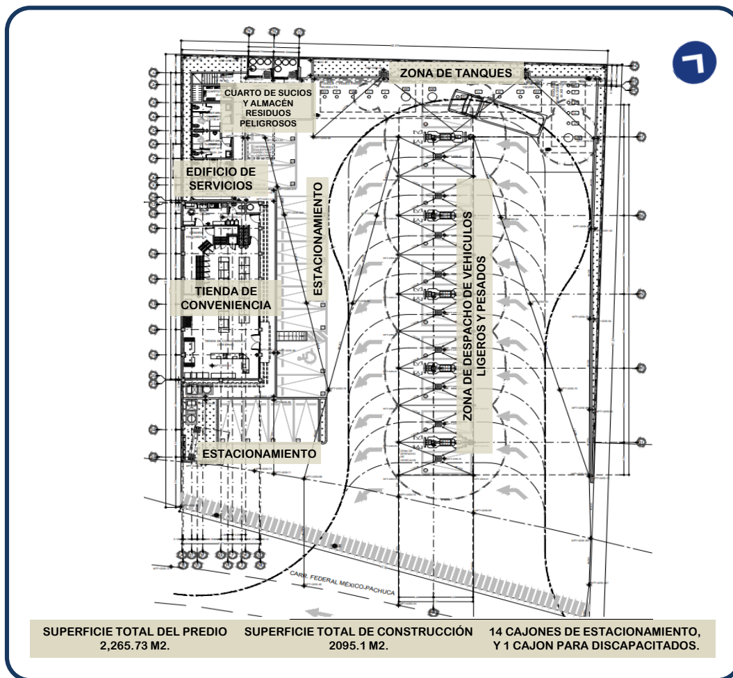
Figura 21 Conjunto arquitectónico
