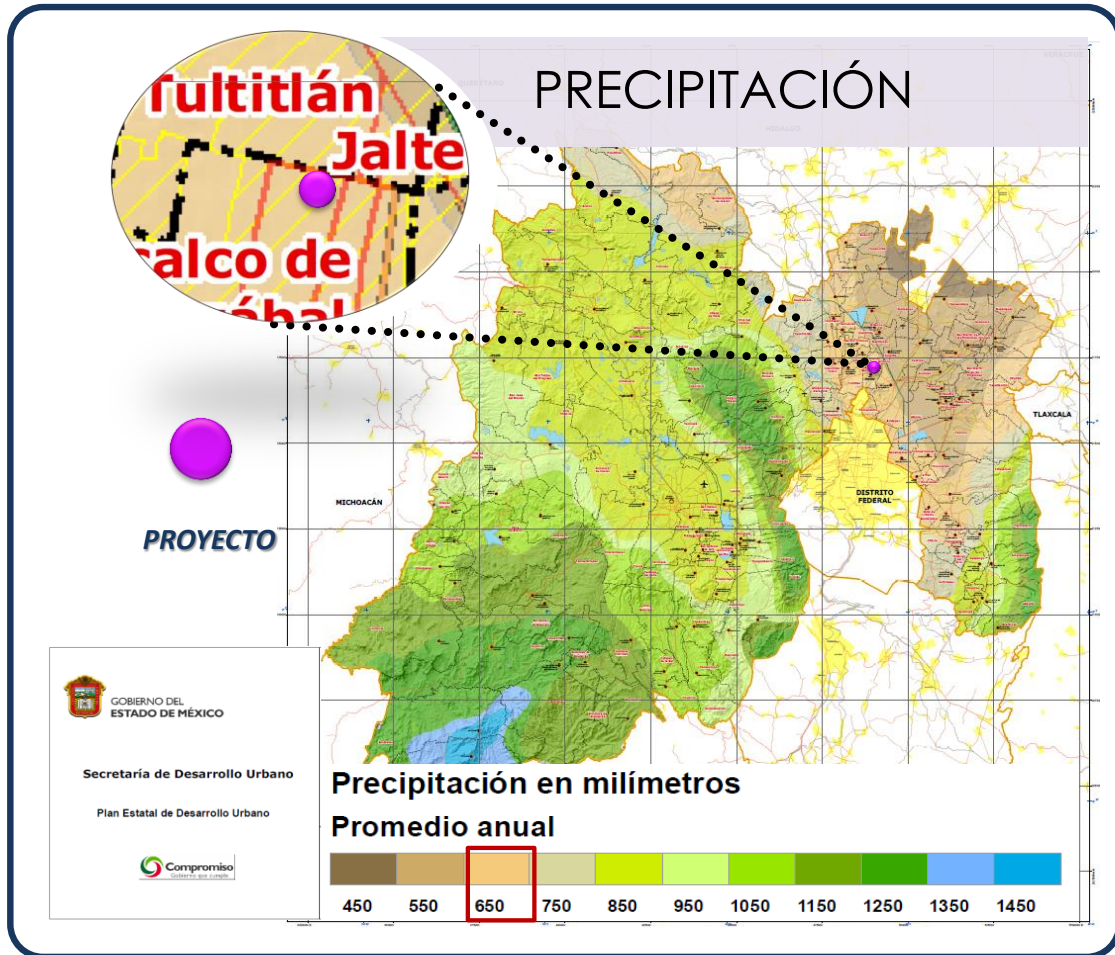
Figura 41 Precipitación promedio
