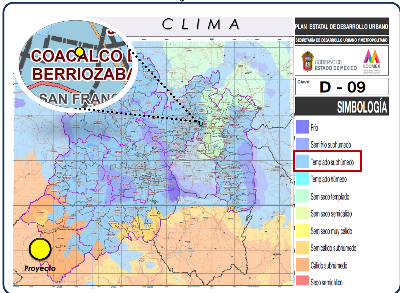
Figura 36 Clima
