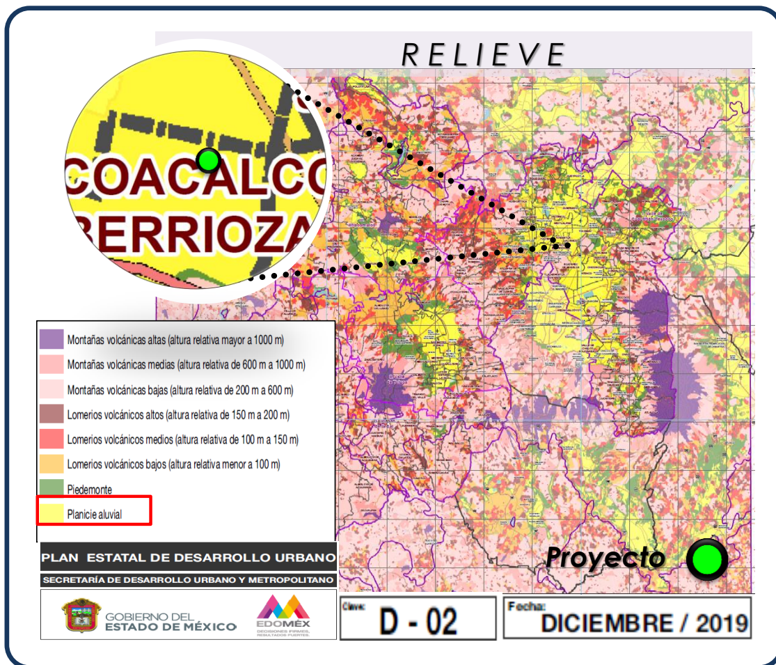
Figura 44 Relieve
