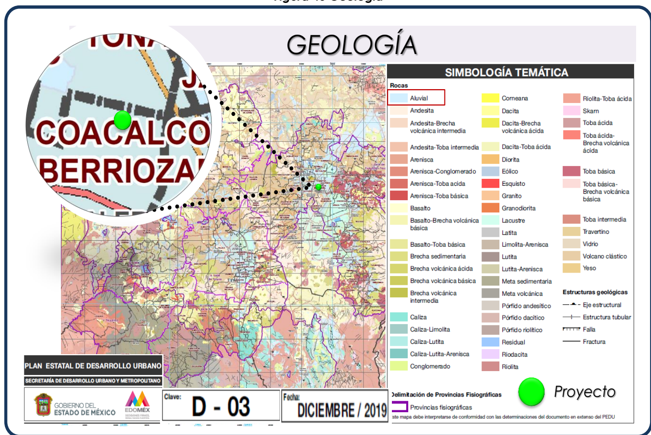
Figura 43 Geología
