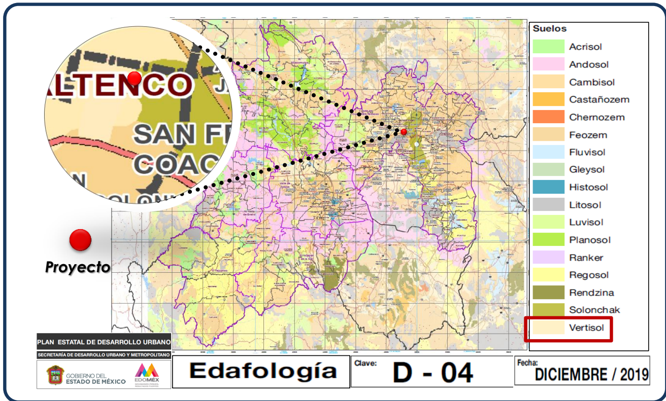
Figura 49 Suelos Dominantes
