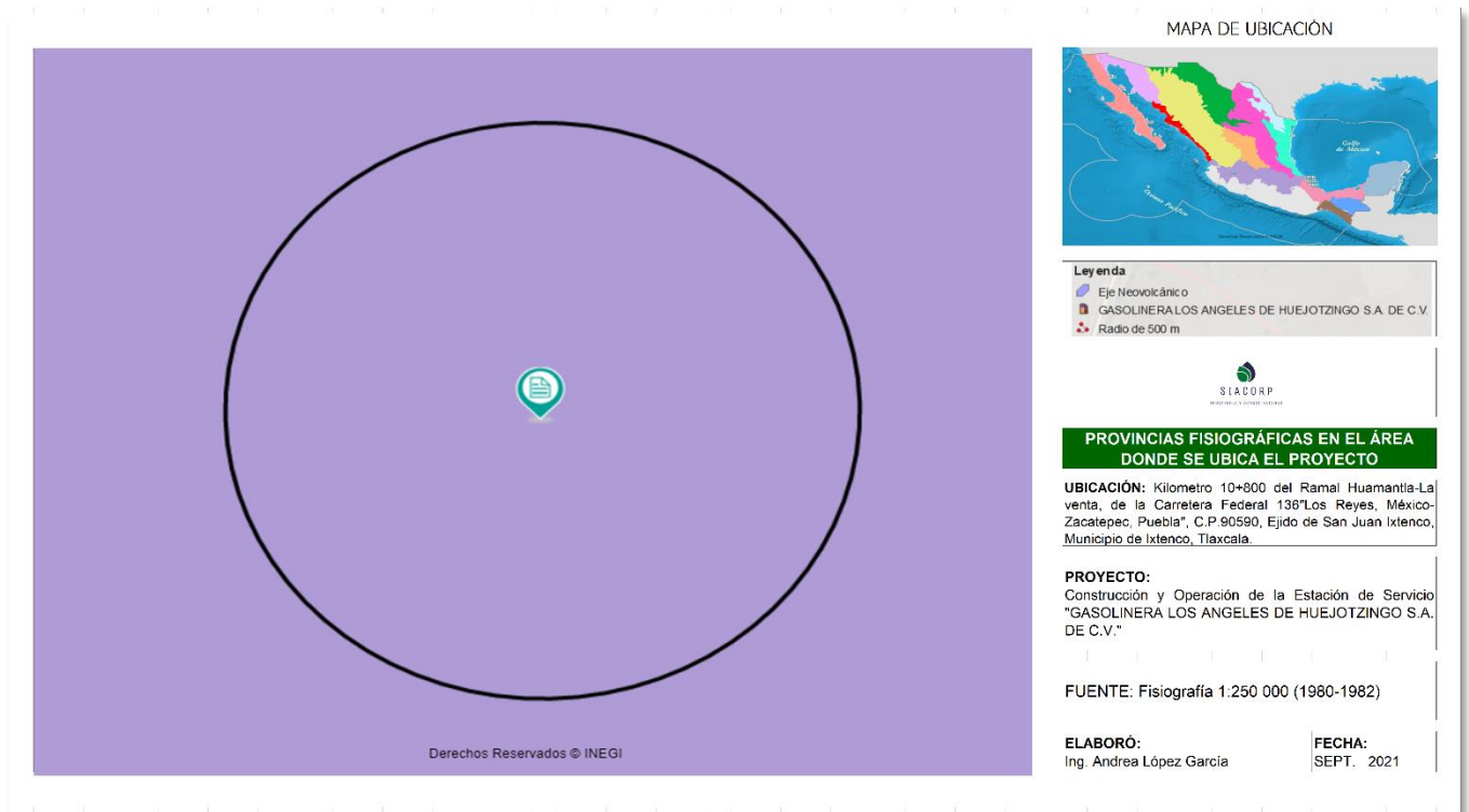
Figura 13. Provincias fisiográficas
