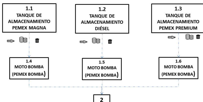
Figura 12. Diagrama de funcionamiento de almacenamiento de combustible.
