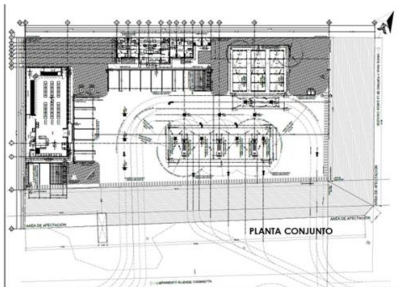
Plano 1. Plano de la estación de servicio.
