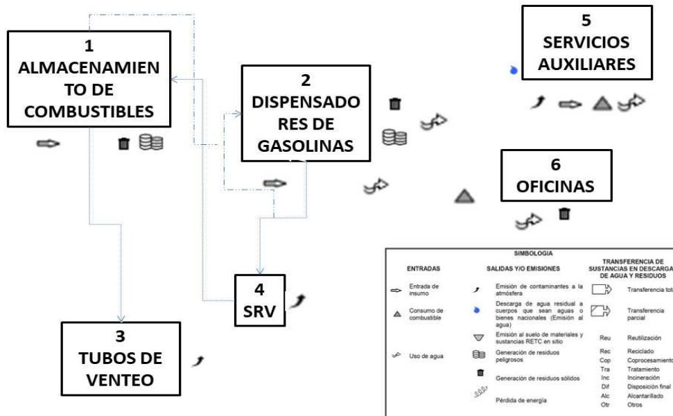
Figura 7. Diagrama de funcionamiento general de la Estación de Servicio.
