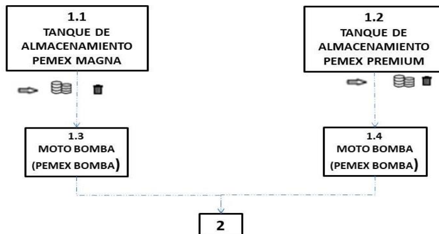
Figura 8. Diagrama de funcionamiento de almacenamiento de combustible.
