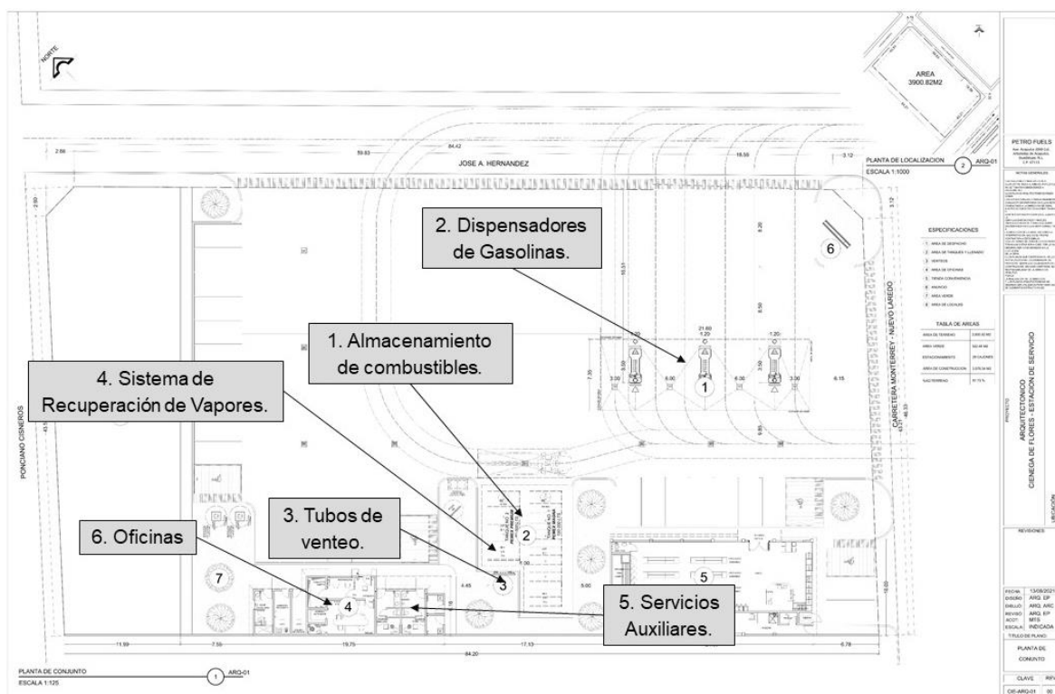
Figura 6. Diagrama de plano.
