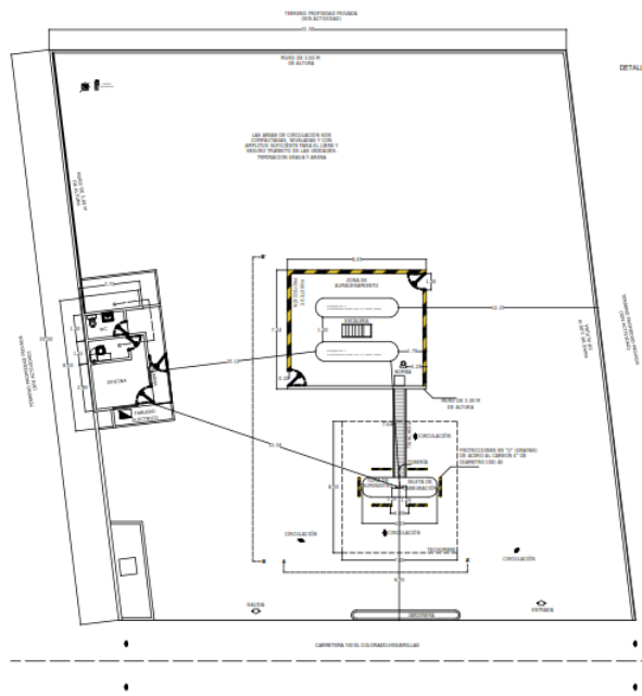
Figura III.1.b)-2. Plano Proyecto Civil
