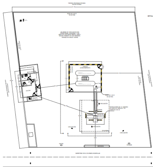
Figura I.1.2.-2. Plano Proyecto Civil
