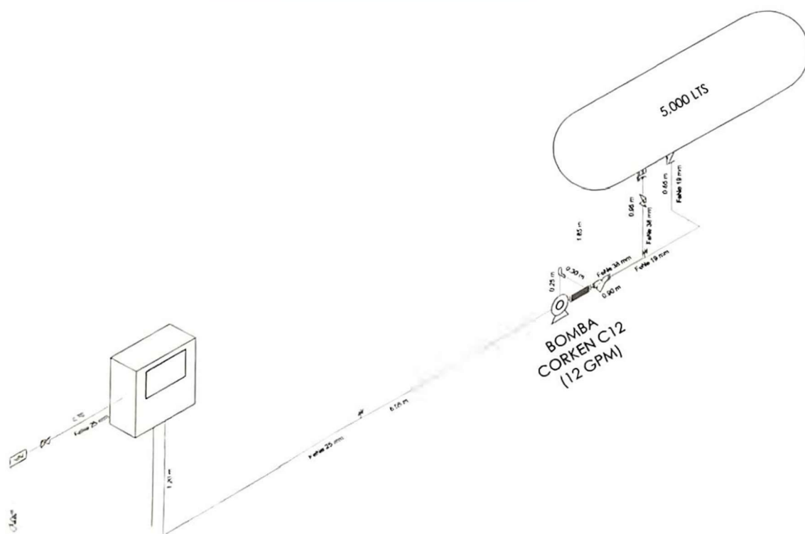
Plano Mecánico del proyecto de la Estación de Gas L.P. para carburación
