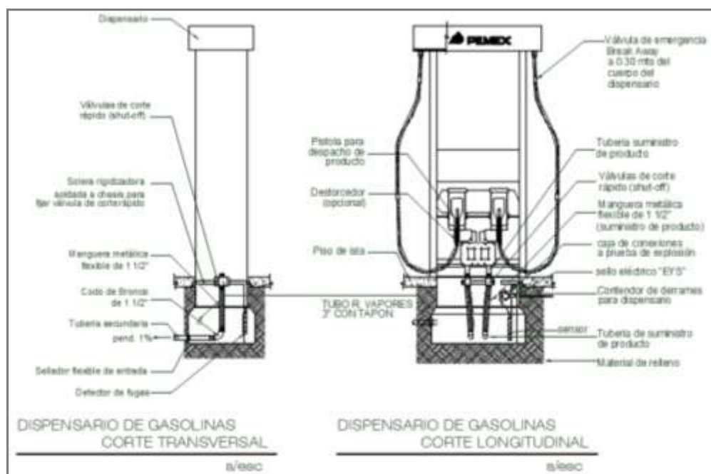
Figura 16. Accesorios de Dispensarios
