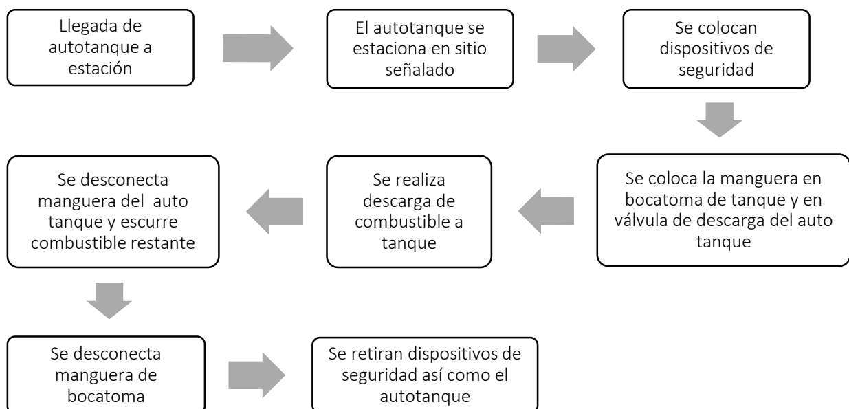
Figura 17. Recepción y descarga de combustibles
