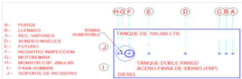
Figura 15. Elementos del tanque de almacenamiento
