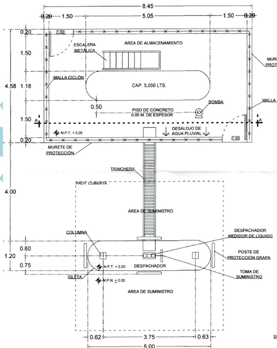
Plano Civil del proyecto de la Estación de Gas L.P. para carburación
