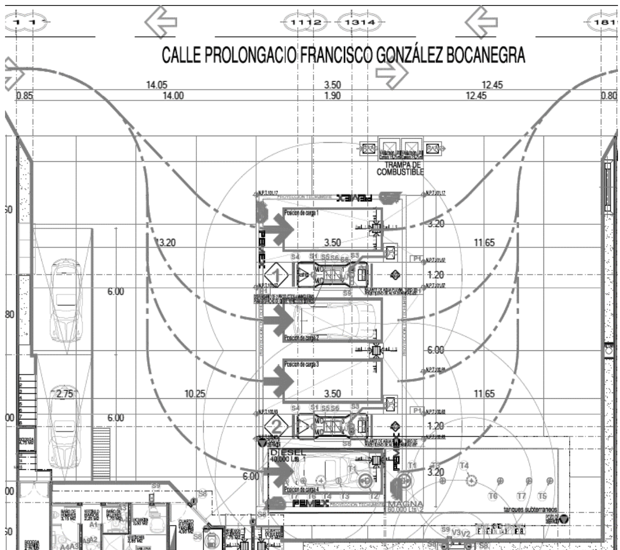
Imagen 8. Plano arquitectónico.
