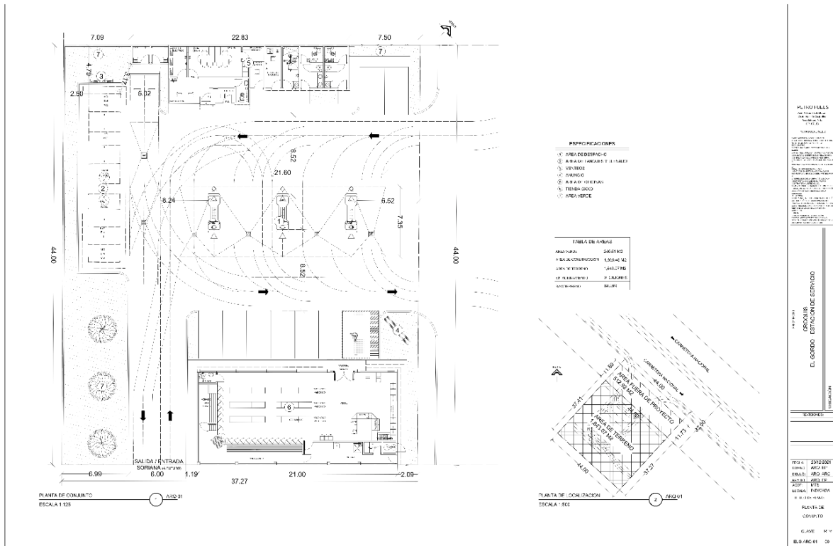
Figura 3. Plano de la estación de servicio.
