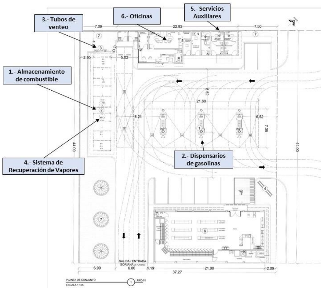
Figura 12. Diagrama de plano.
