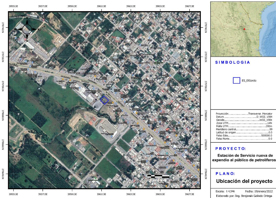
Figura 2. Plano de ubicación y colindancias.
