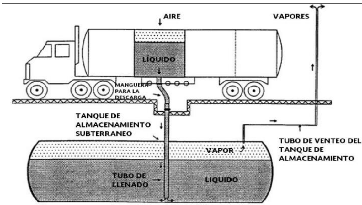
Figura 16. Punto de emisión llenado de tanque estacionario.
