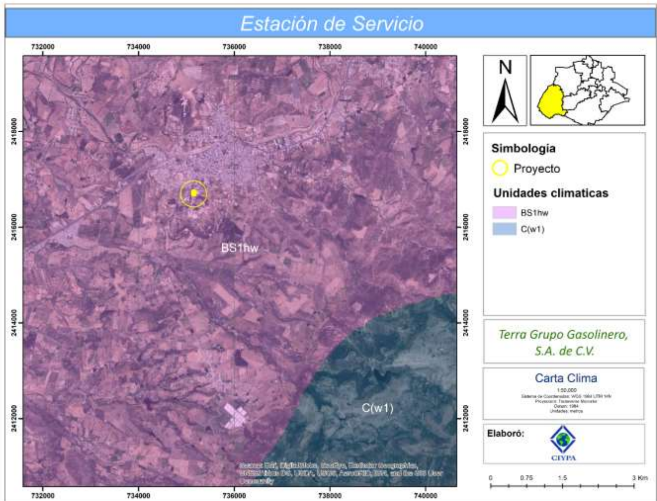
Figura 23. Carta Clima
