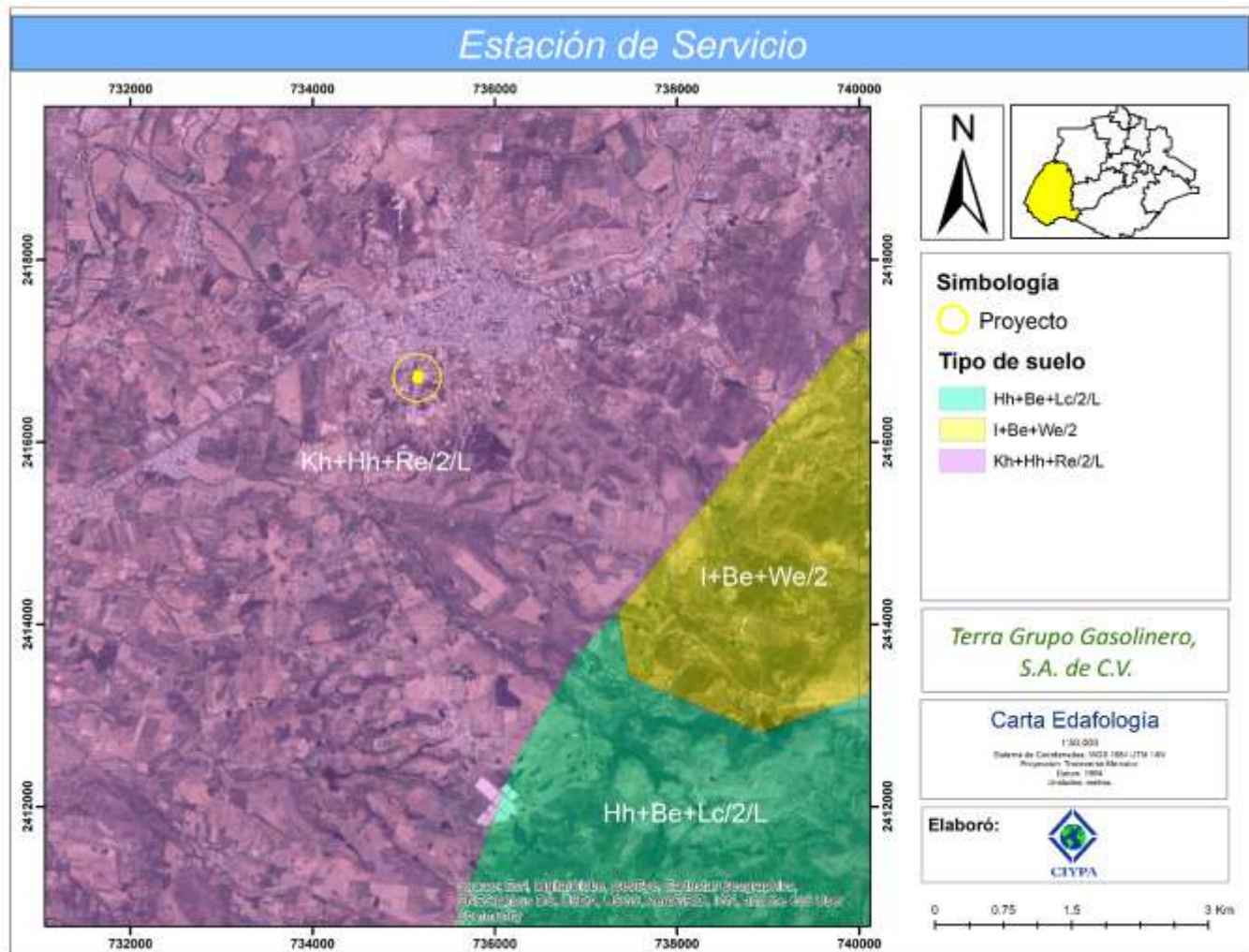
Figura 28. Carta Edafología
