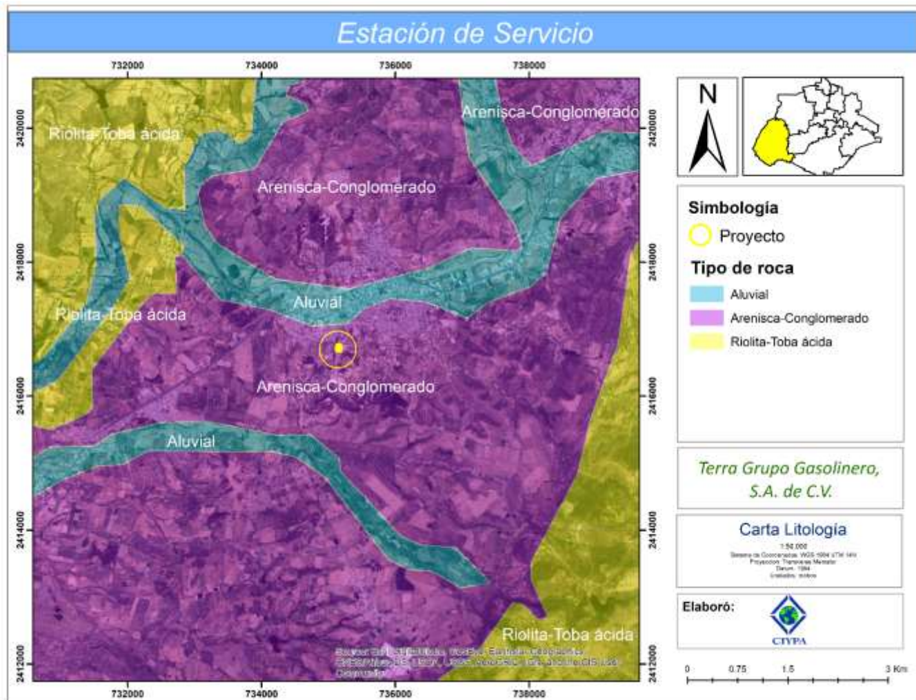
Figura 24. Carta Litología
