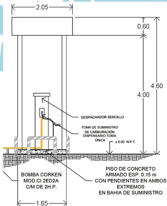
Imagen 11. Vista Longitudinal de la Toma de Suministro.
