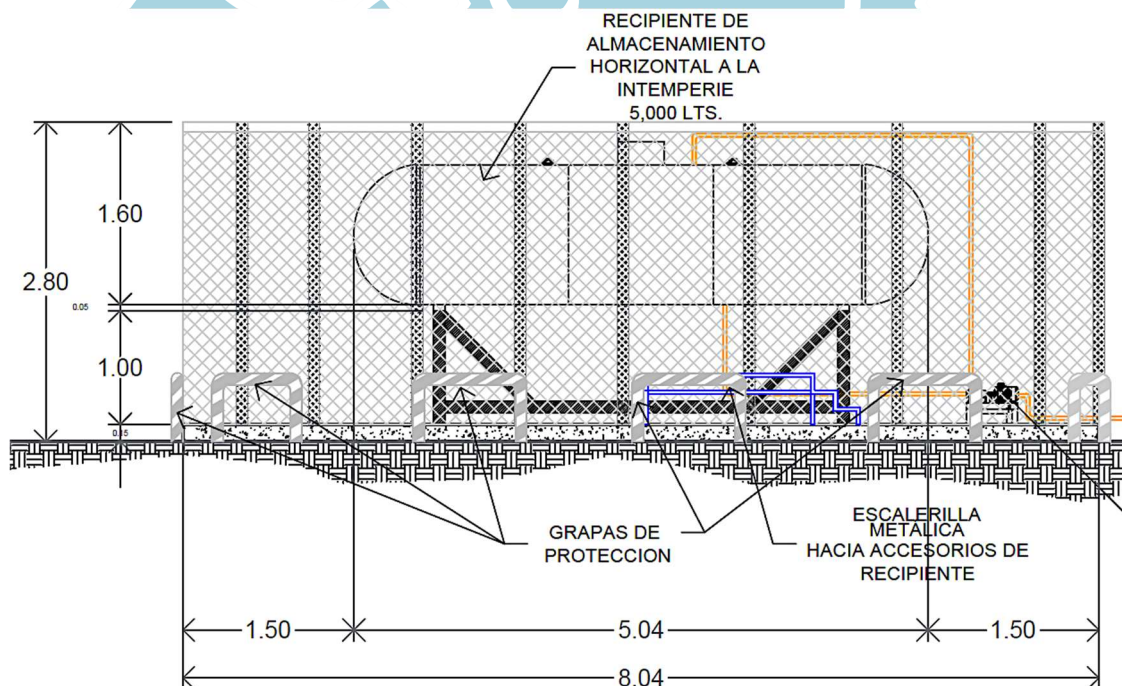
Imagen 10. Vista Longitudinal del Tanque de Almacenamiento.
