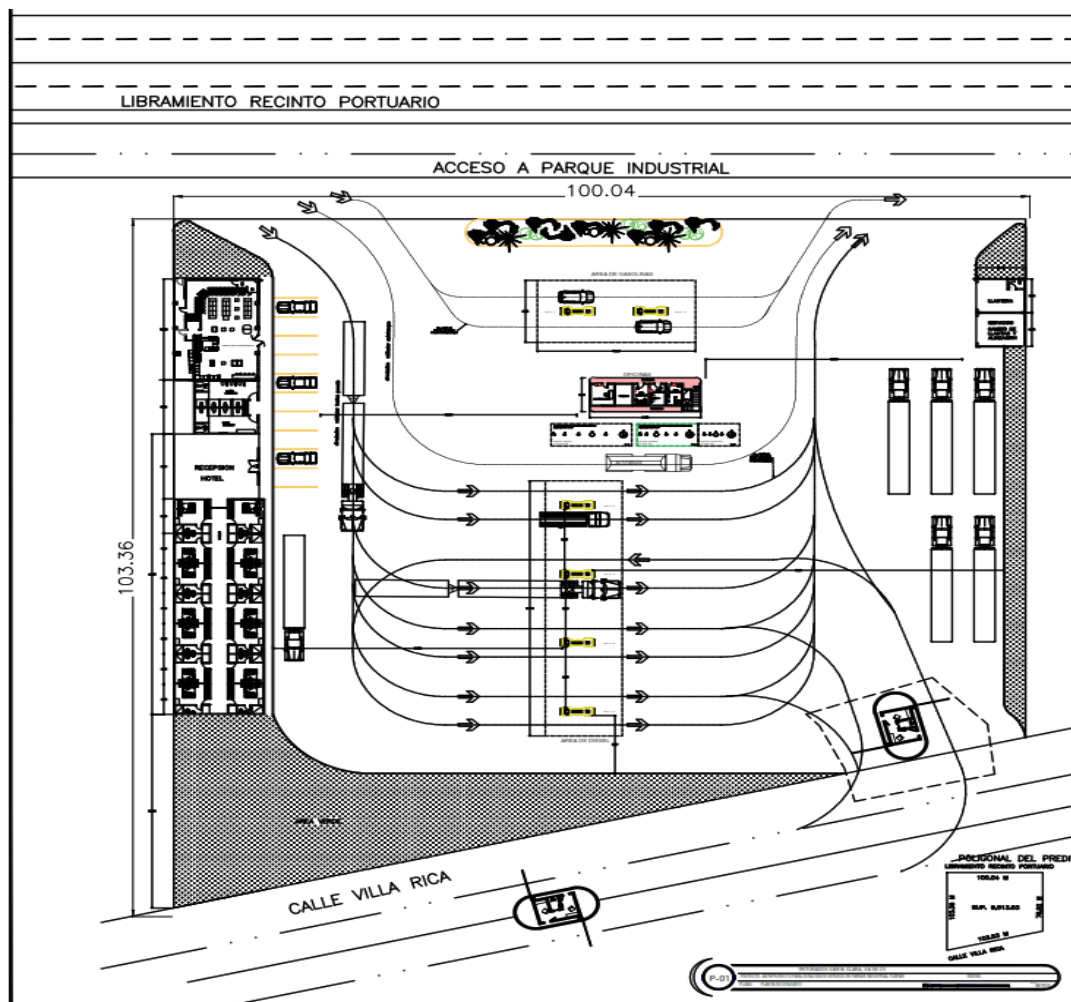
Imagen 8. Plano arquitectónico.
