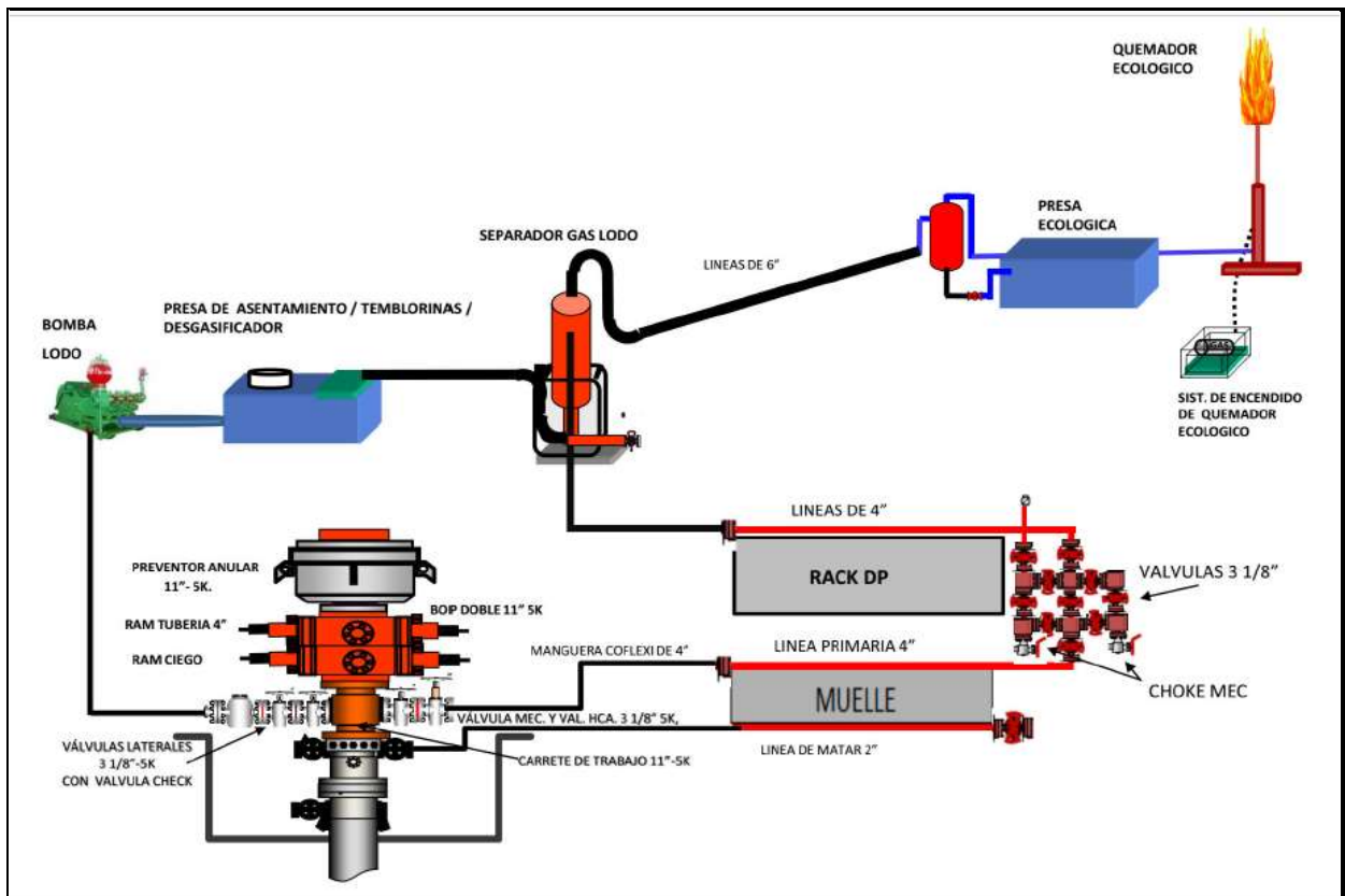
Figura III.1.2.5.3-2.- Diagrama de instalación del equipo de control superficial en fase 6 ¾”.
