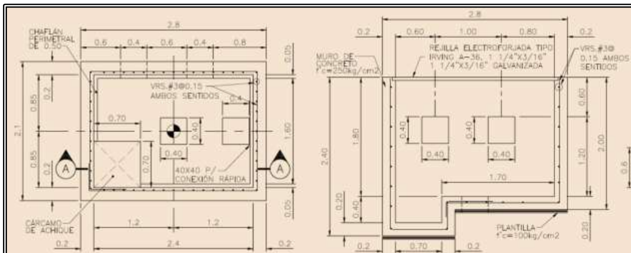
Figura III.1.2.3-1.- Diseño del contrapozo.
