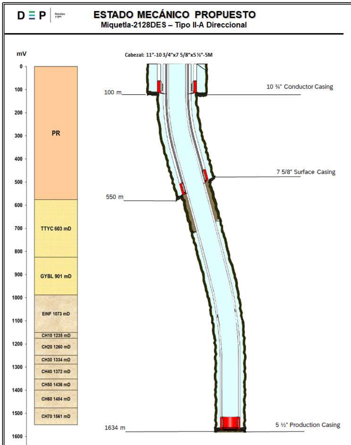
Figura III.1.2.5-1.- Esquema mecánico propuesto.
