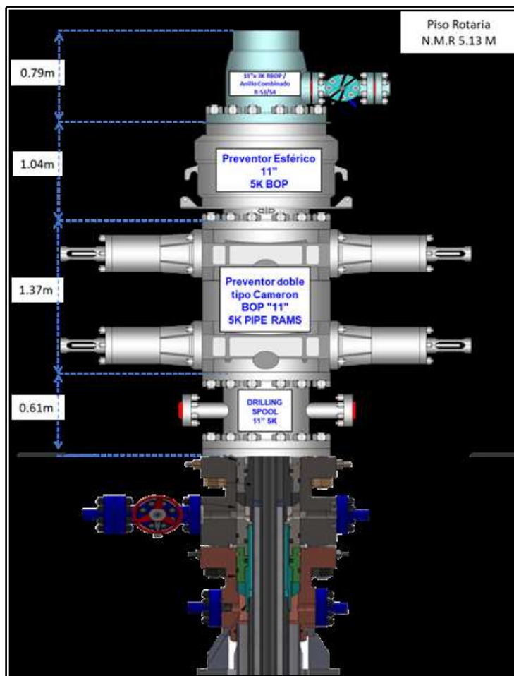
Figura III.1.2.5.3-1.- Conjunto de preventores para la fase 6 \frac{3}{4} ".
