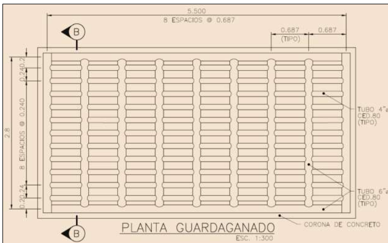
Figura III.1.2.2-2.- Diseño del guardagando.
