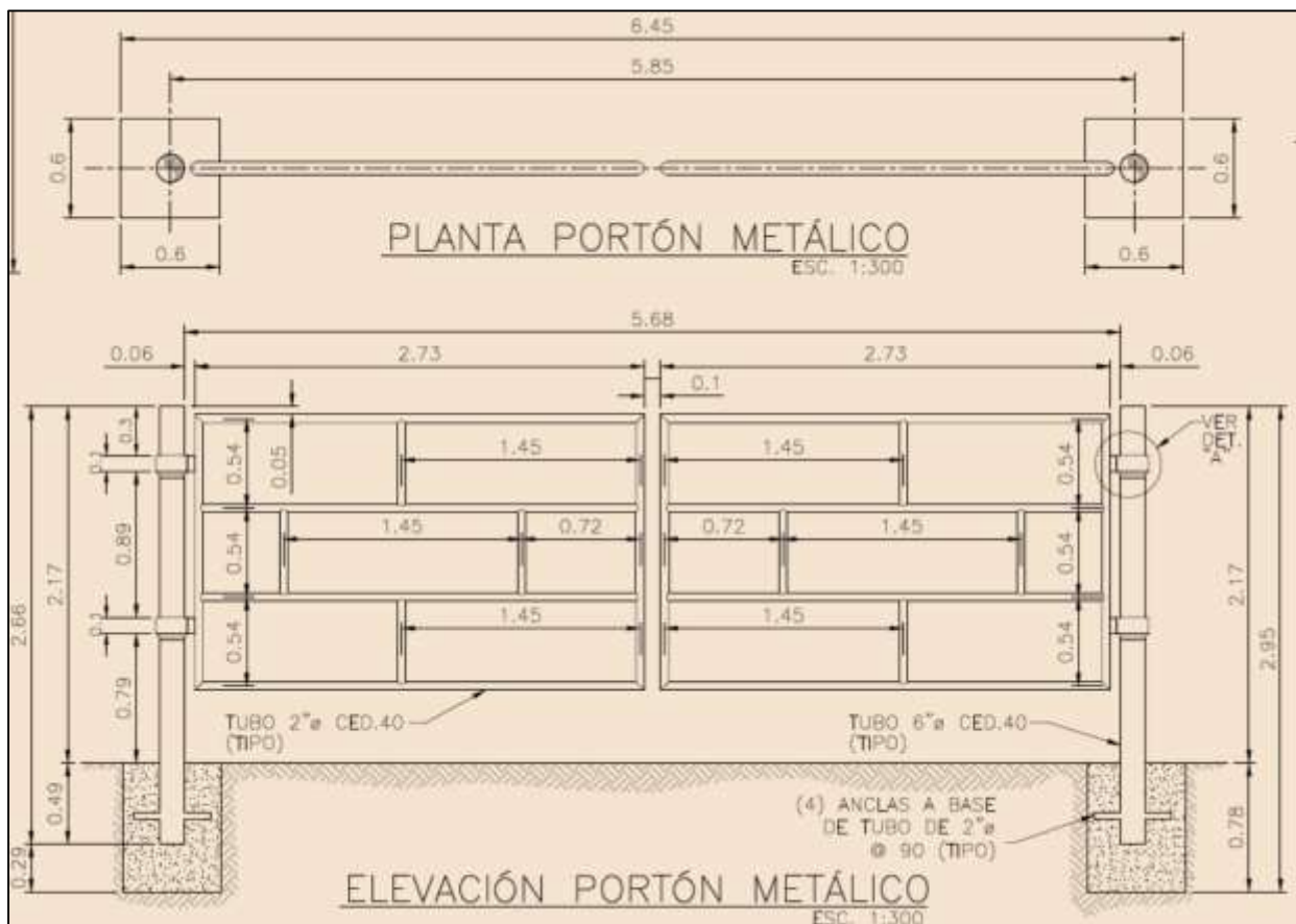
Figura III.1.2.2-2.- Diseño del portón metálico.
