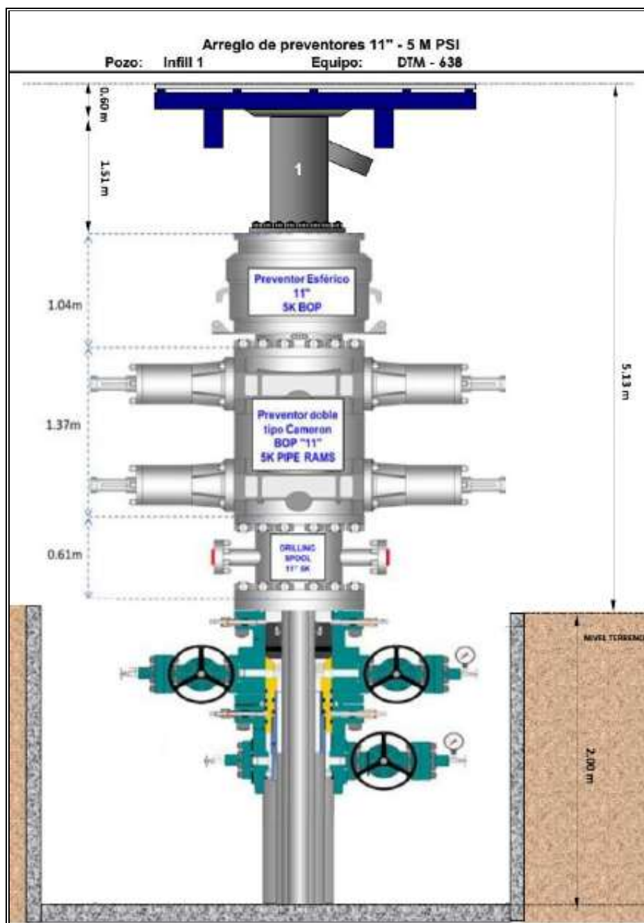
Figura III.1.2.5.3-1.- Conjunto de preventores para la fase 6 ¾".
