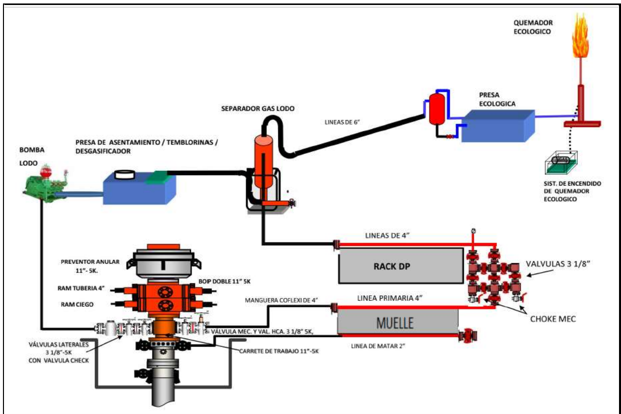
Figura III.1.2.5.3-2.- Diagrama de instalación del equipo de control superficial en fase 6 3/4.
