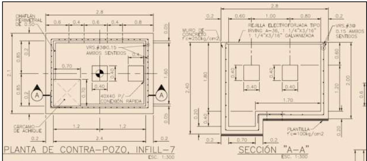
Figura III.1.2.3-1.- Diseño del contrapozo.
