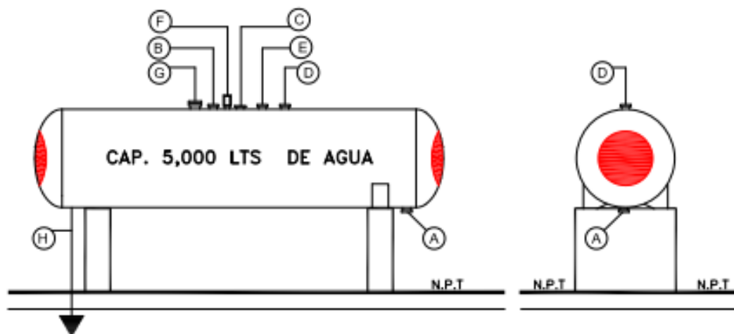
Figura 9. Instrumental de seguridad del tanque de almacenamiento.
