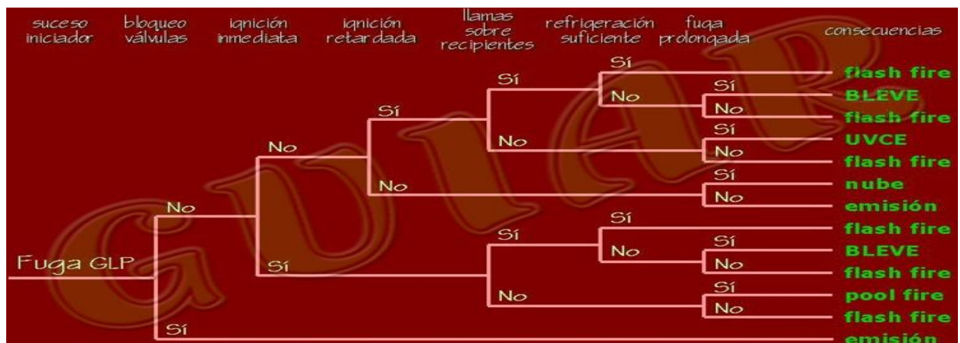
Figura 15. Árbol de sucesos para fuga de gas L.P. en zona próxima al tanque de almacenamiento.
