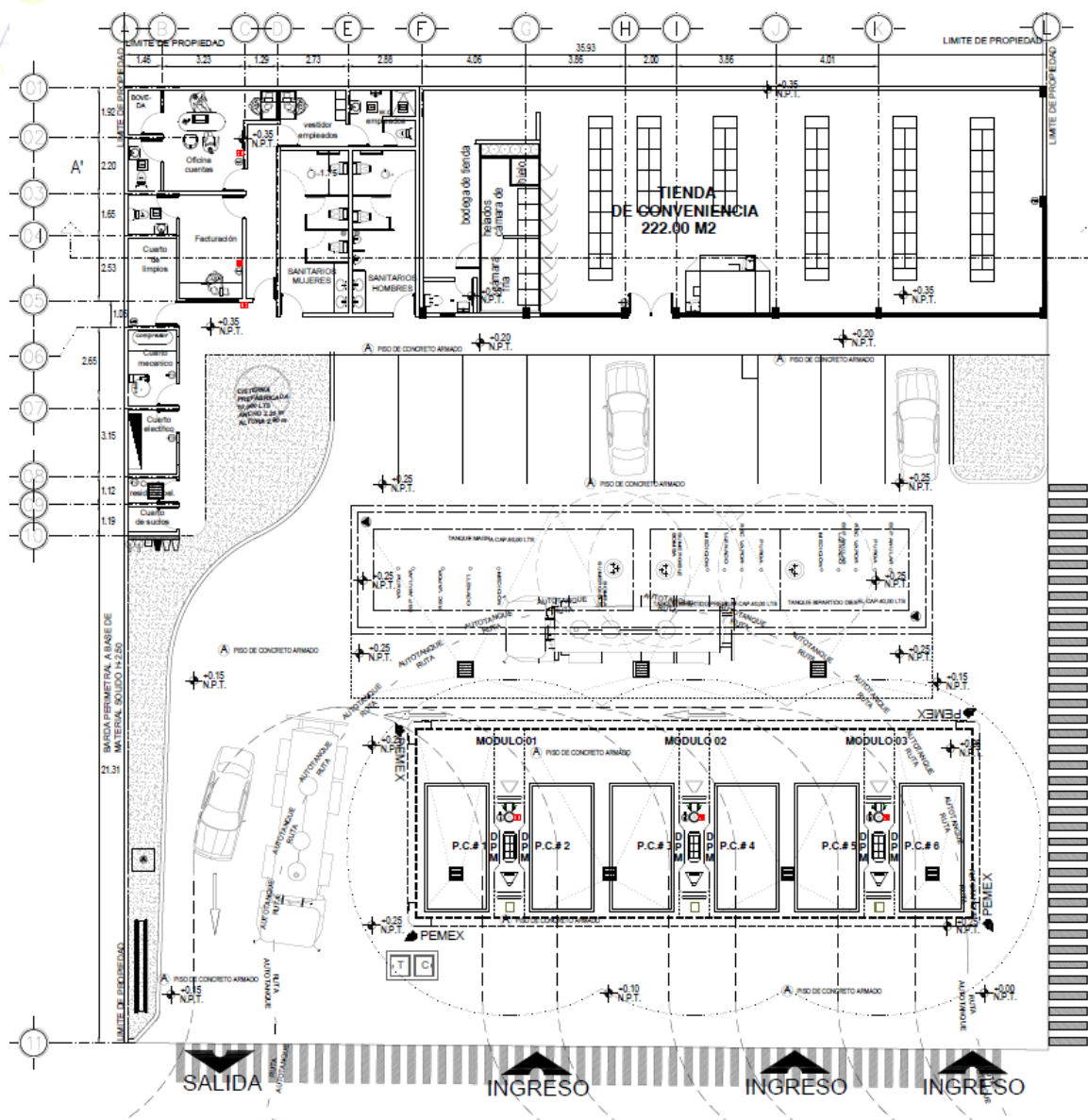
Imagen 12. Plano de Conjunto de COMERCIALIZADORA DE HIDROCARBUROS AMEZGOM S.A. DE C.V.
