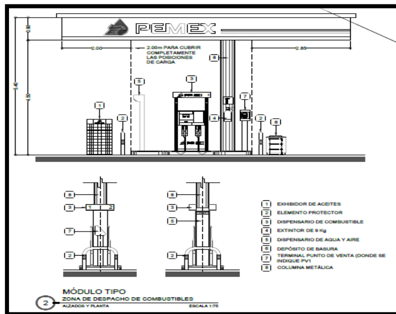
Imagen 11. Diagrama Tipo del Módulo de Abastecimiento.
