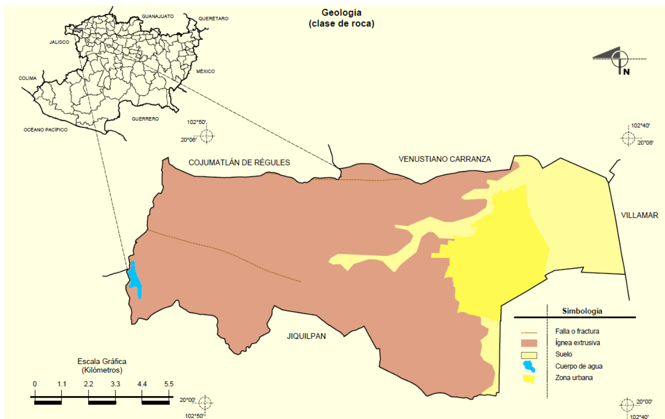
Figura 9.- Geología del Área de influencia
