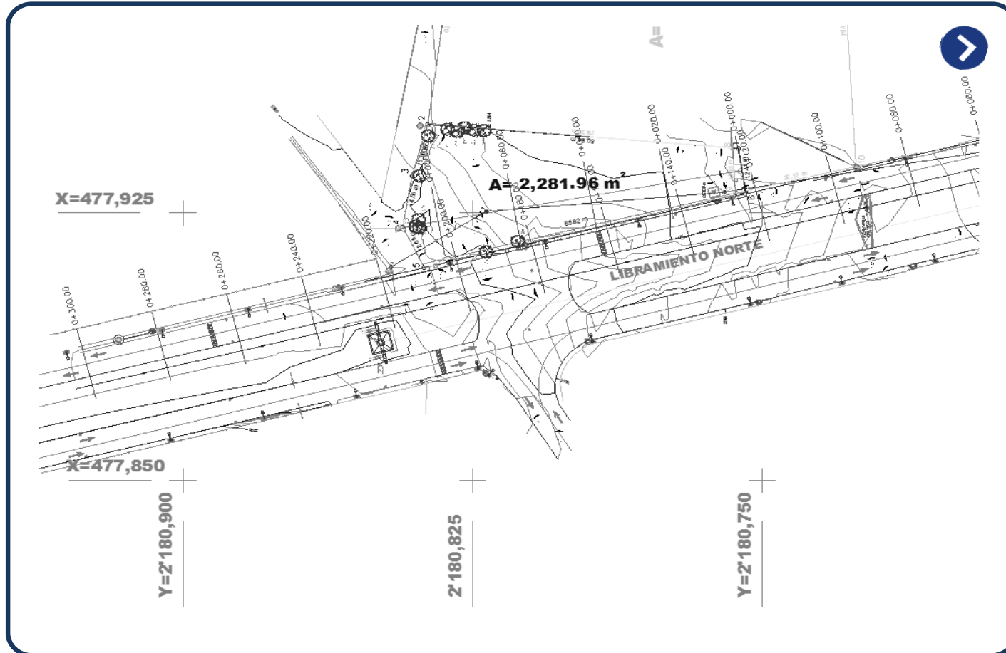
Figura 18 Plano Topográfico
