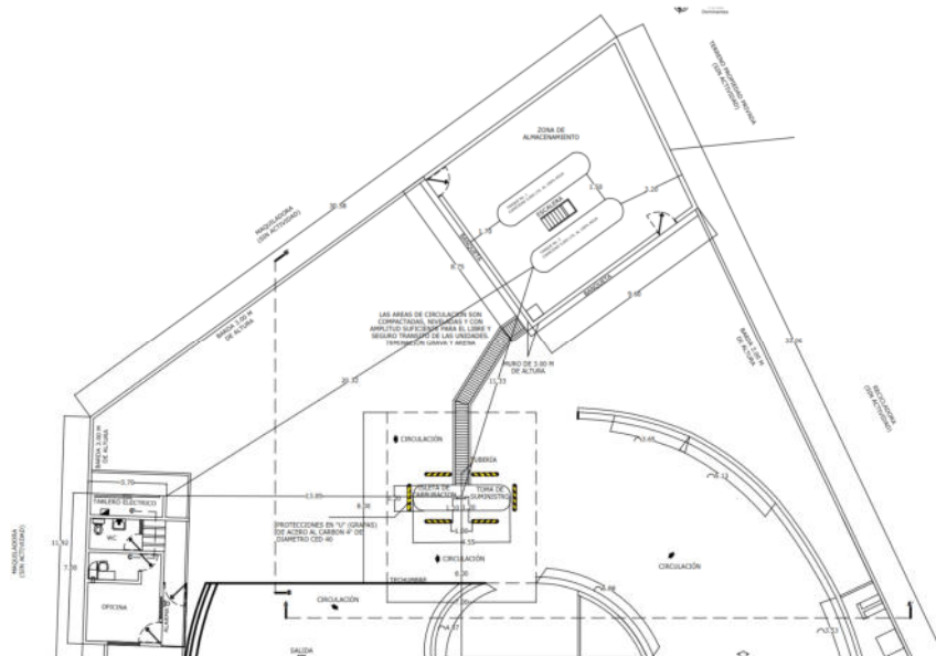
Figura III.1.b)-2. Plano Proyecto Civil
