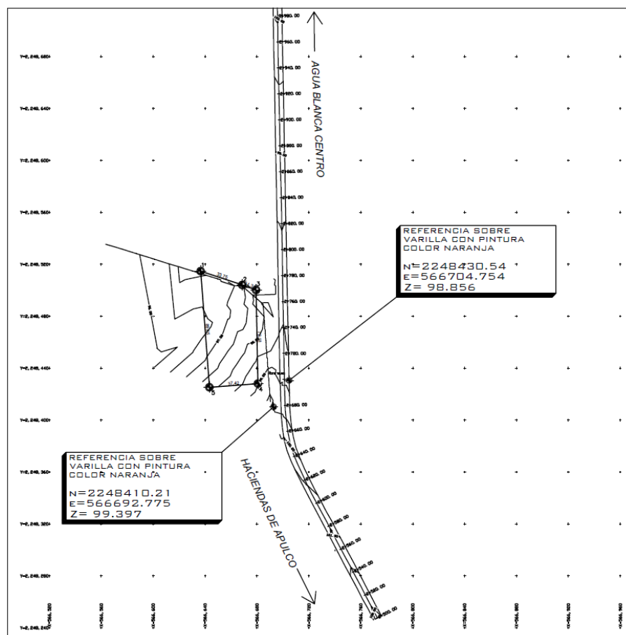
Plano Topográfico
